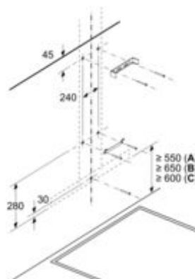
Rozměry v mm Hloubka nástěnného panelu
