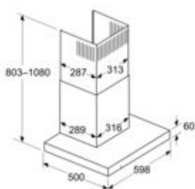
Rozměry v mm Recirkulační systém
