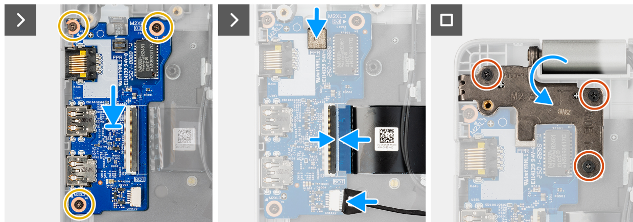
Obrázek 52. Vložení desky I/O
