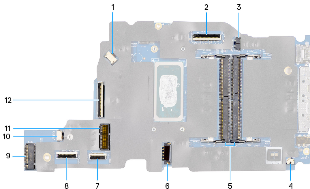
Obrázek 72. Konektory na základní desce
