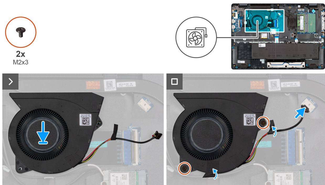
Obrázek 34. Montáž ventilátoru
