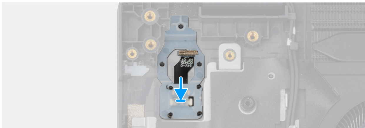
Obrázek 56. Montáž vypínače se čtečkou otisků prstů
