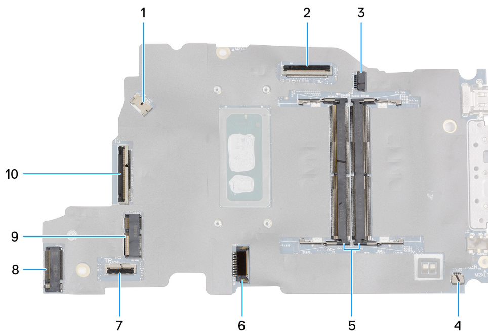
Obrázek 60. Konektory na základní desce
