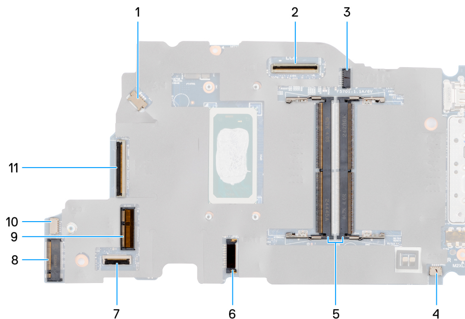
Obrázek 66. Konektory na základní desce
