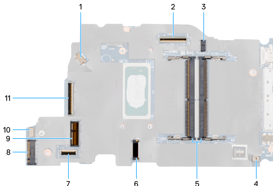
Obrázek 63. Konektory na základní desce
