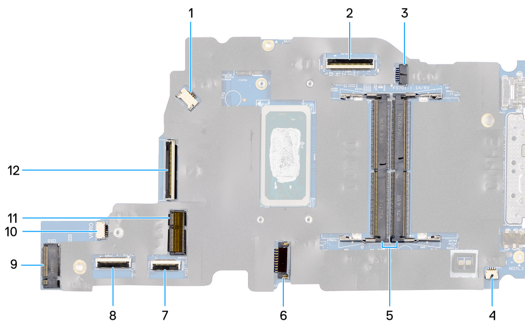
Obrázek 69. Konektory na základní desce
