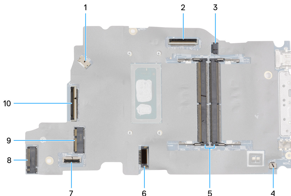
Obrázek 57. Konektory na základní desce
