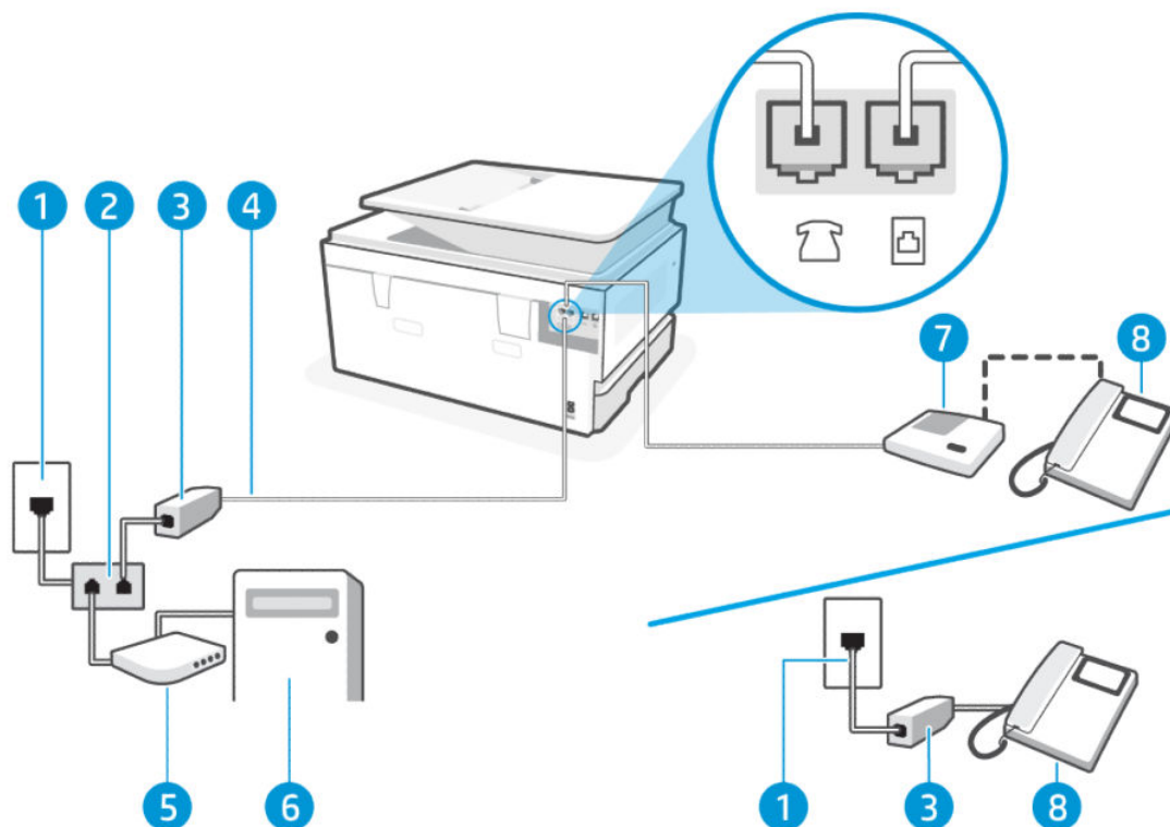
Tabulka 7-15 Pohled zezadu na tiskárnu
