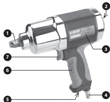
3. ábra - A WI 680 típusú ütvecsavarozó részei
