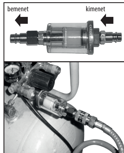
11. ábra - Szűrő (leválasztó) csatlakoztatása.
