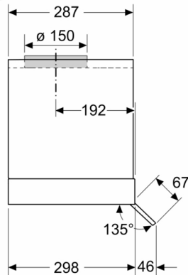
Rozměry v mm Boční pohled
