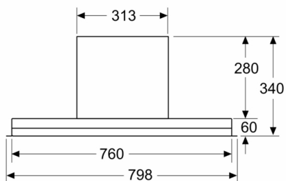
Rozměry v mm Čelní pohled
