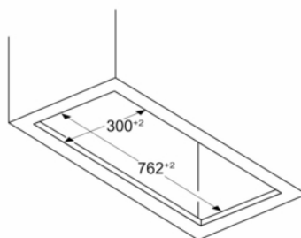
Rozměry v mm Příklad instalace do výřezu v nábytku
