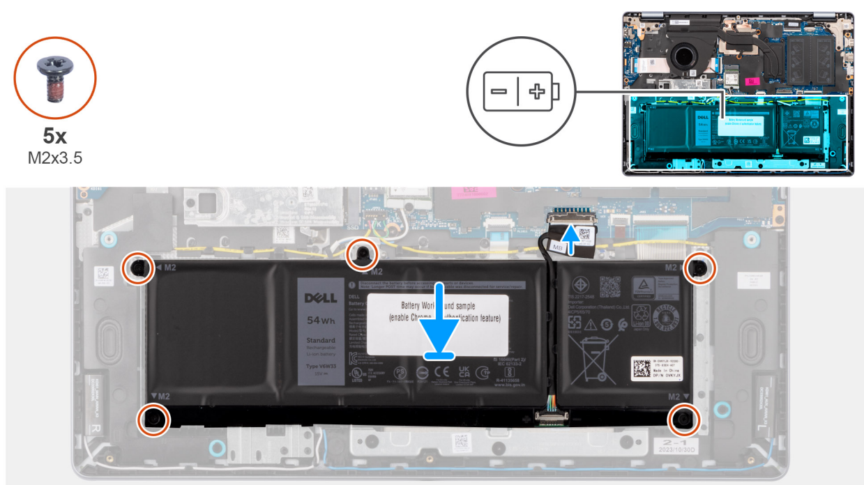
Obrázek 17. Vložení baterie
