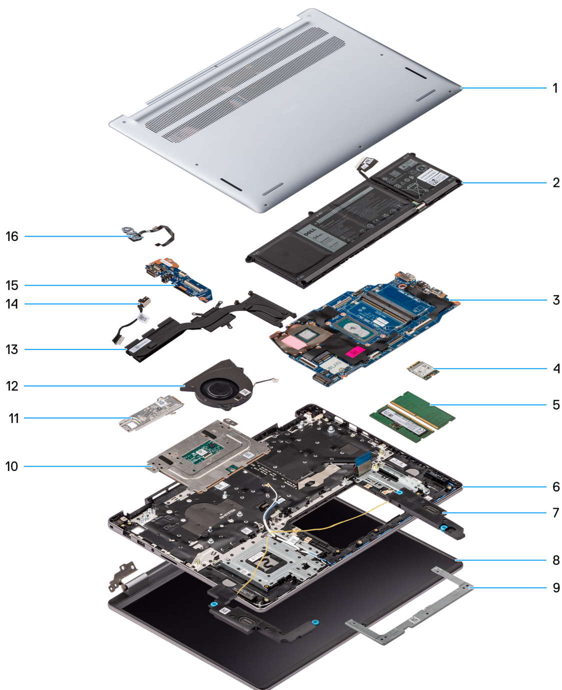
Obrázek 11. Hlavní komponenty počítače Dell 16 DC16251
