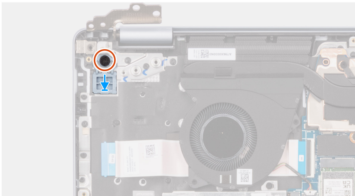
Obrázek 52. Montáž vypínače
