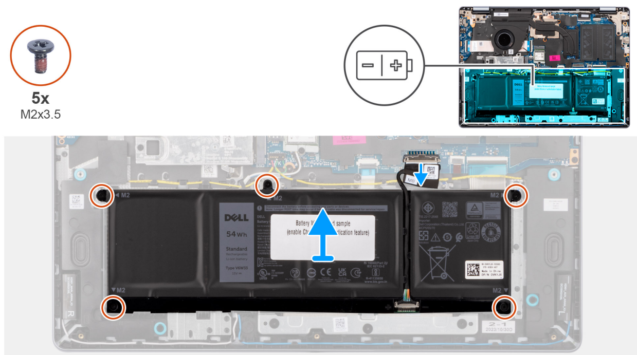
Obrázek 16. Vyjmutí baterie
