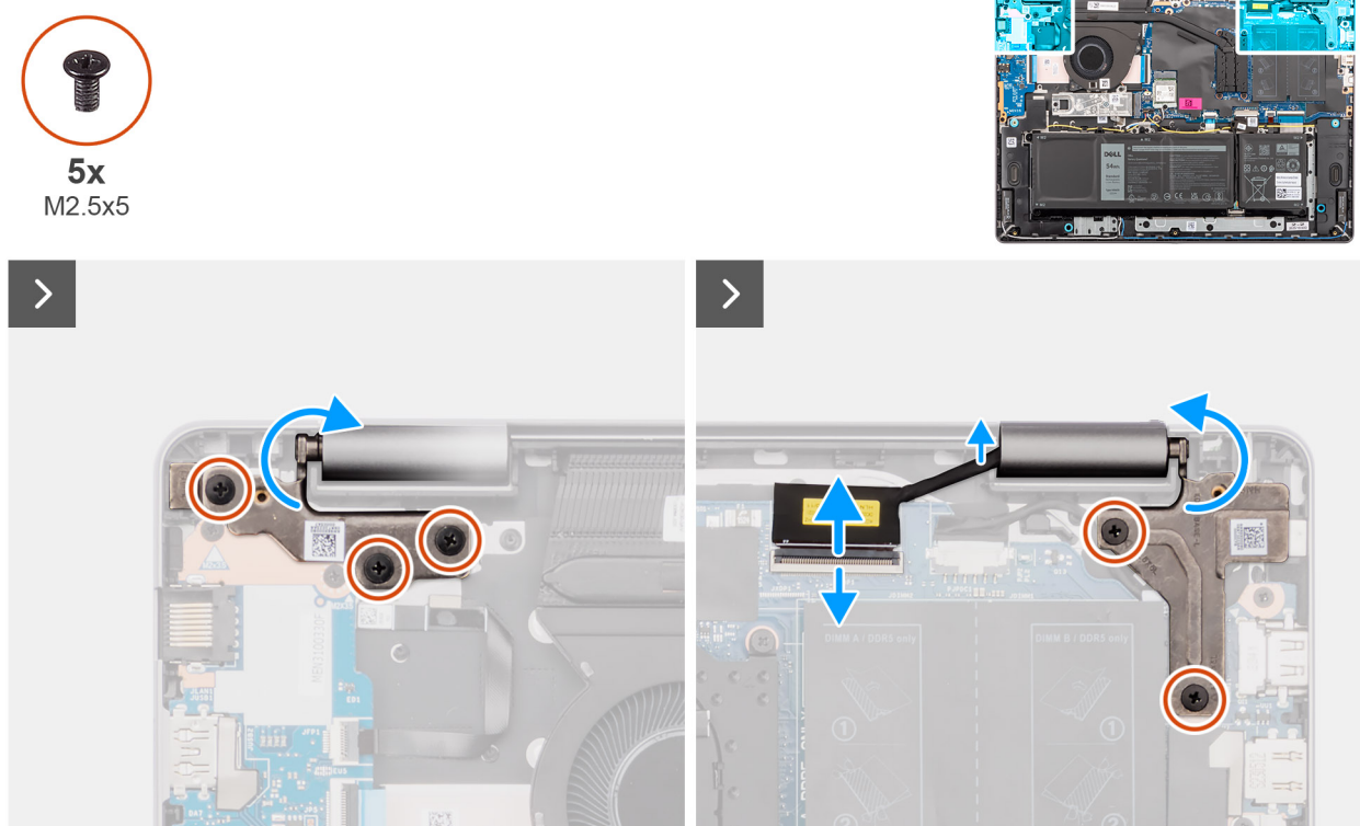
Obrázek 47. Demontáž sestavy displeje
