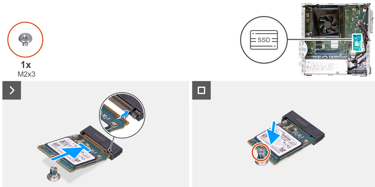
Obrázek 26. Instalace disku SSD M.2 2230
