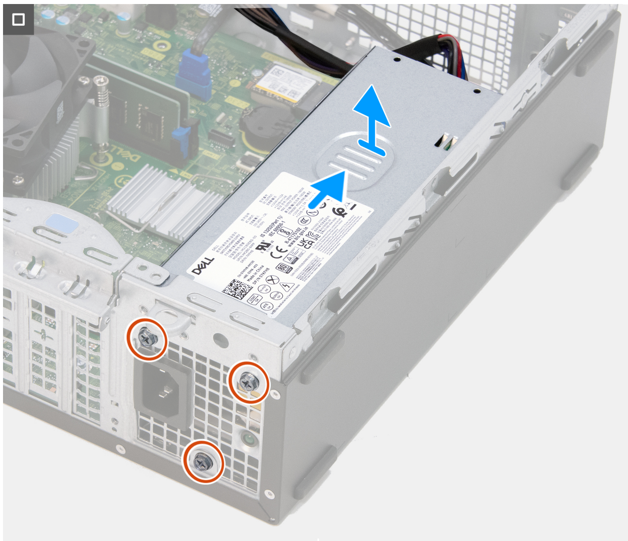
Obrázek 34. Demontáž napájecího zdroje
