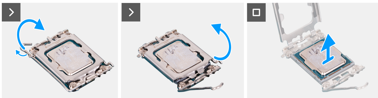
Obrázek 41. Demontáž procesoru
