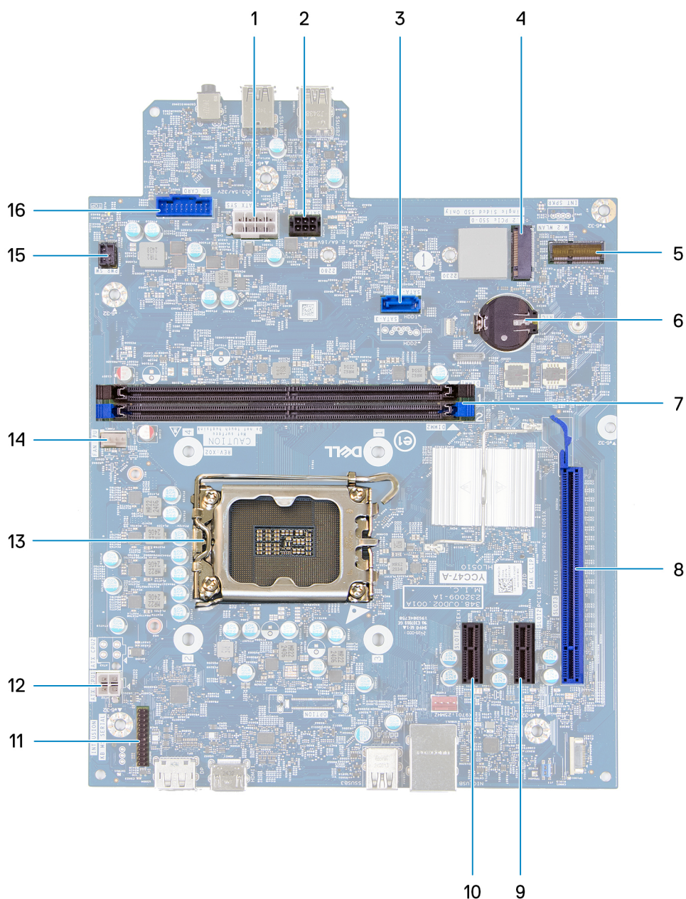
Obrázek 48. Přehled základní desky
