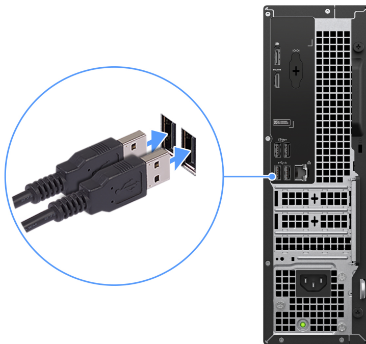
Obrázek 4. Připojení kabelové klávesnice a myši k Dell Pro Slim Essential QVS1260
