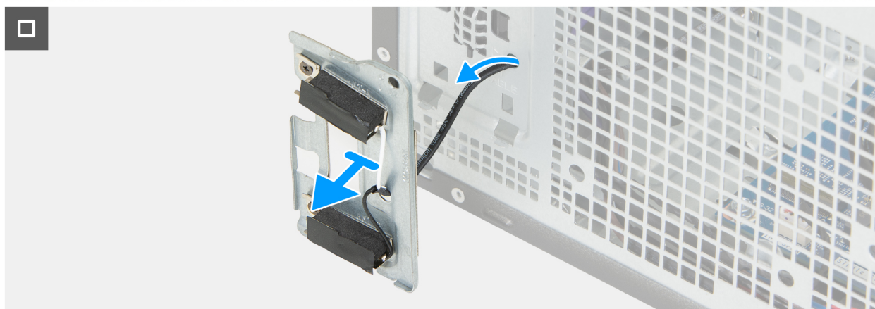
Obrázek 31. Demontáž modulu antény
