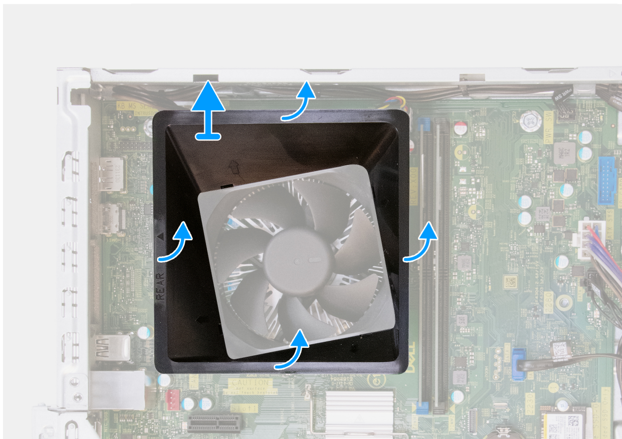
Obrázek 37. Demontáž krytu ventilátoru
