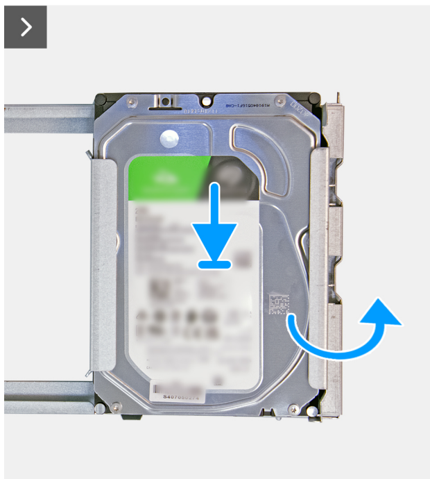
Obrázek 22. Montáž pevného disku
