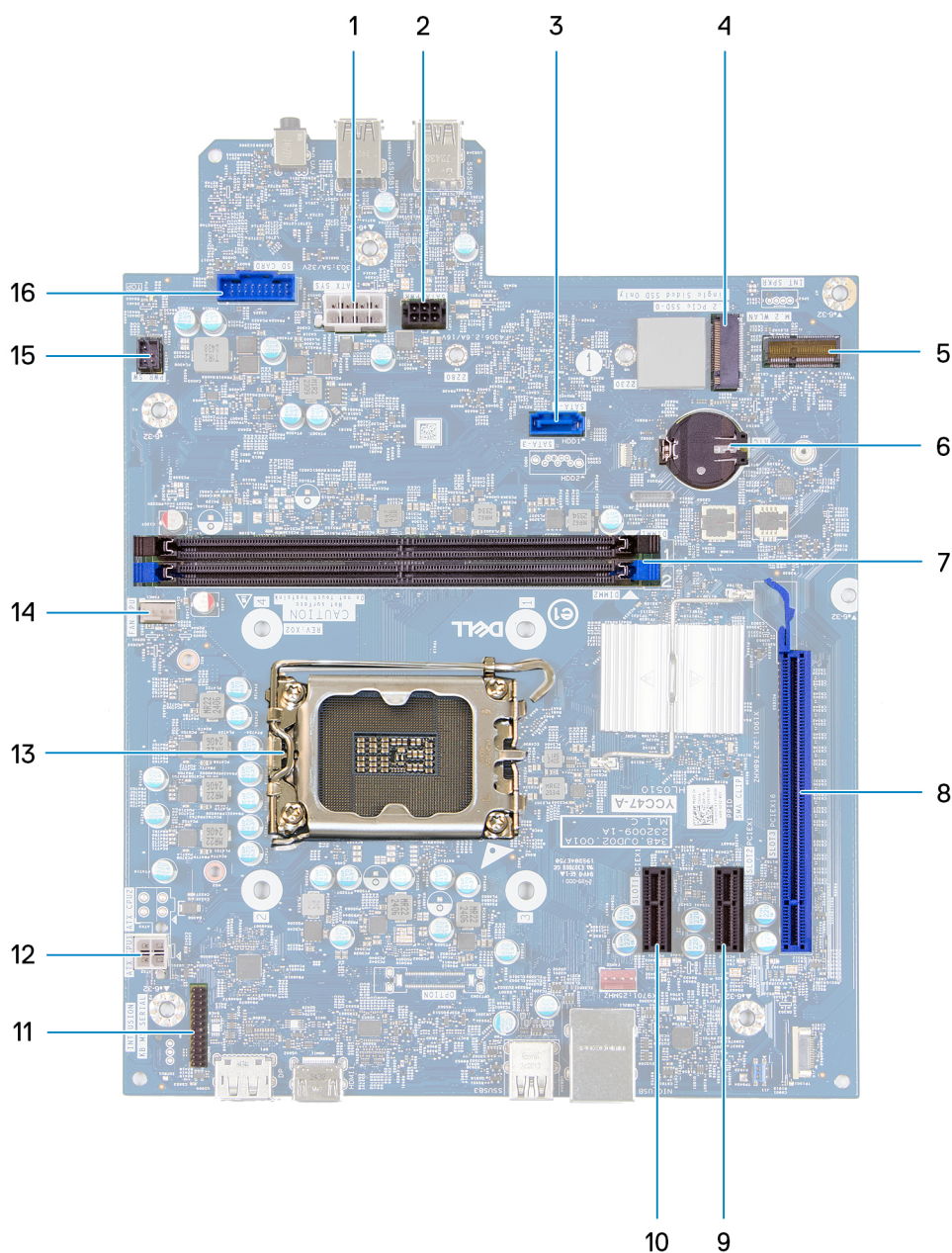
Obrázek 52. Přehled základní desky
