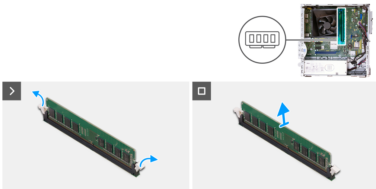
Obrázek 23. Vyjmutí paměťového modulu
