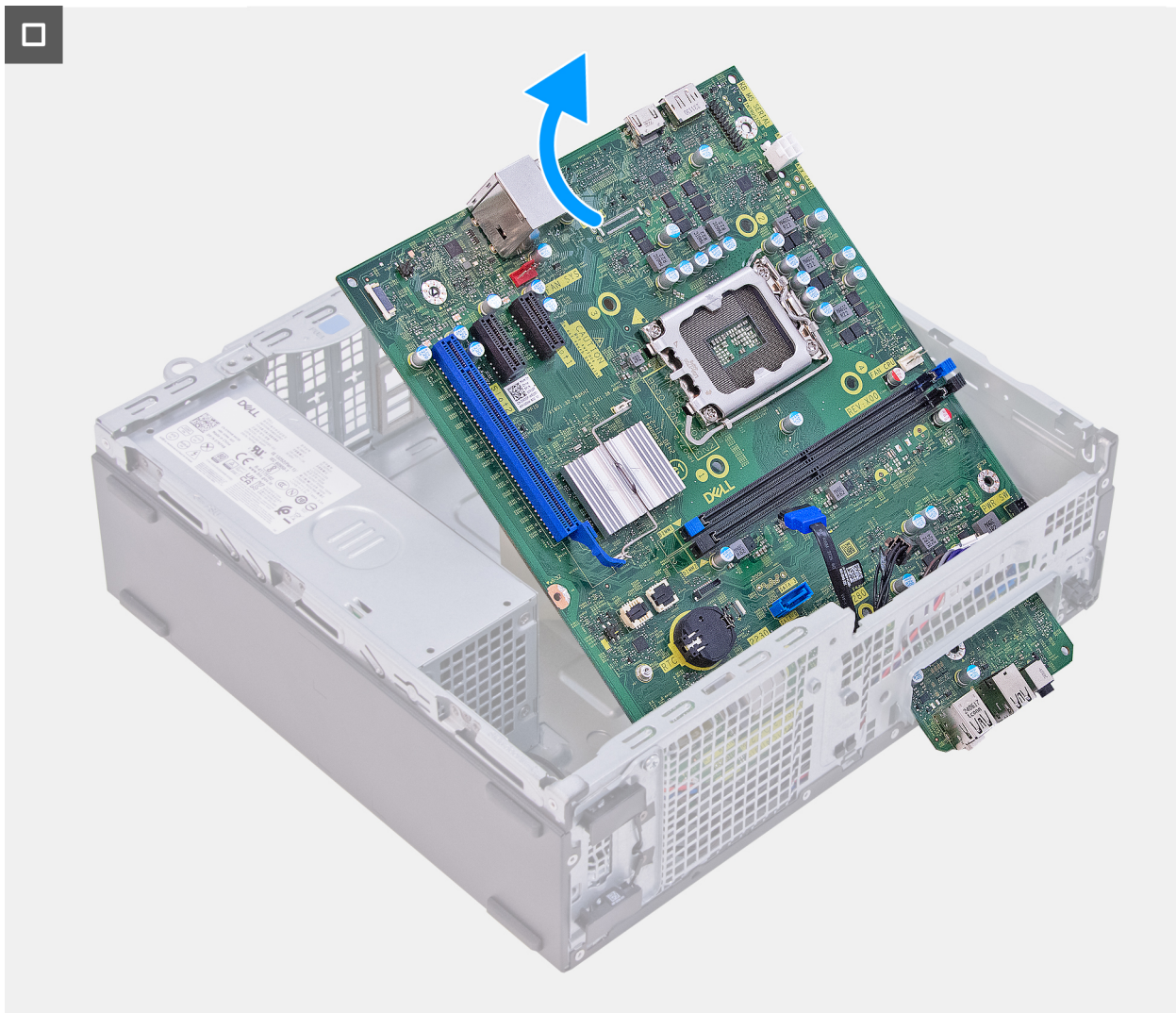
Obrázek 51. Demontáž základní desky
