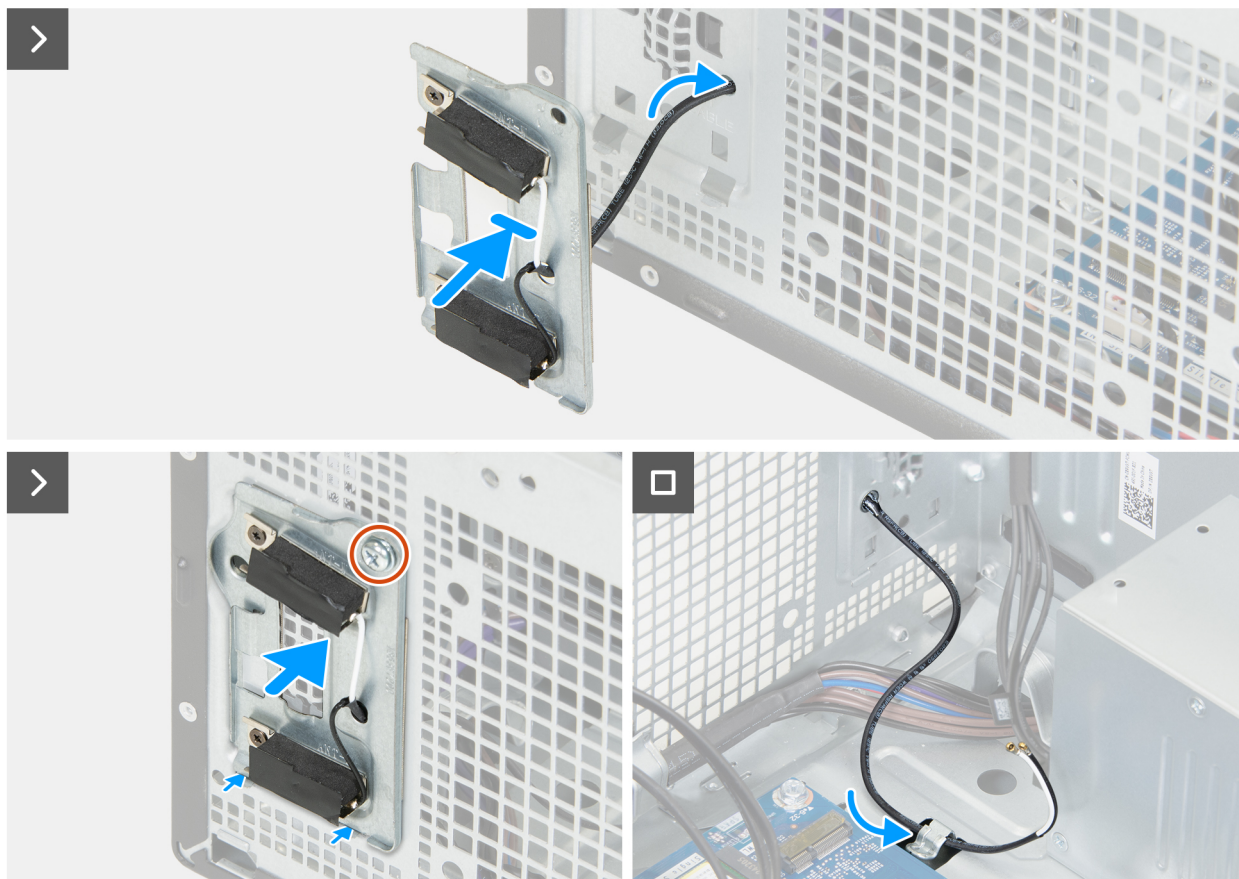
Obrázek 32. Montáž modulu antény
