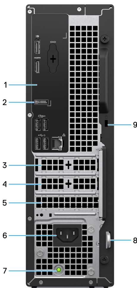
Obrázek 2. Pohled zezadu na tenký Dell Pro Slim Essential QVS1260
