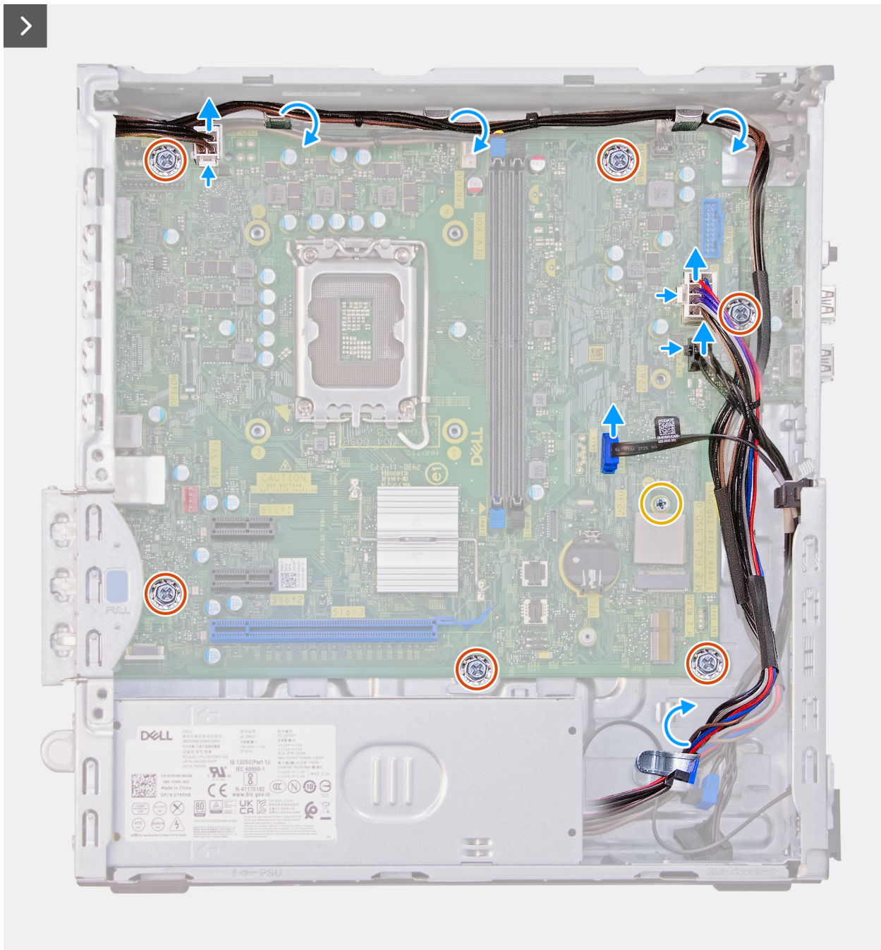
Obrázek 50. Demontáž základní desky
