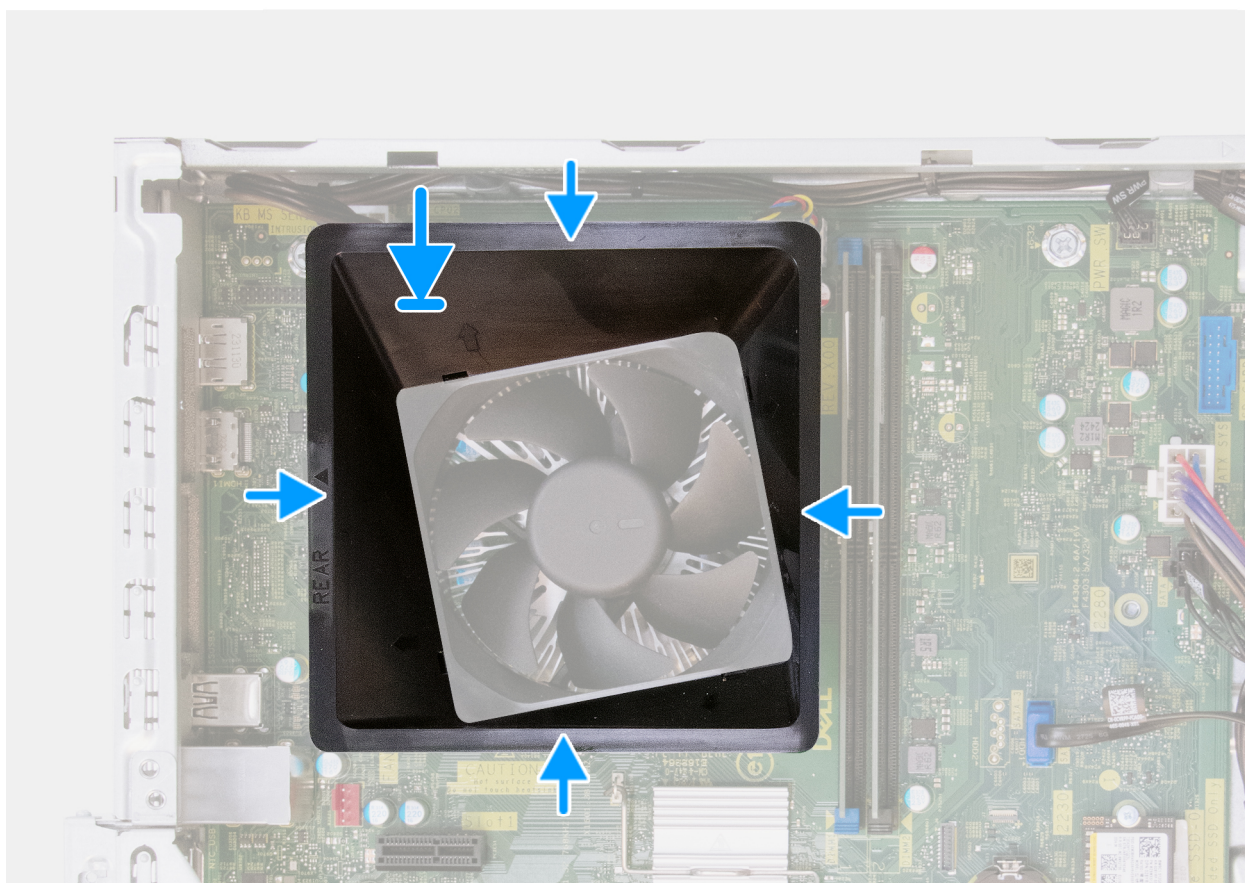
Obrázek 38. Montáž krytu ventilátoru
