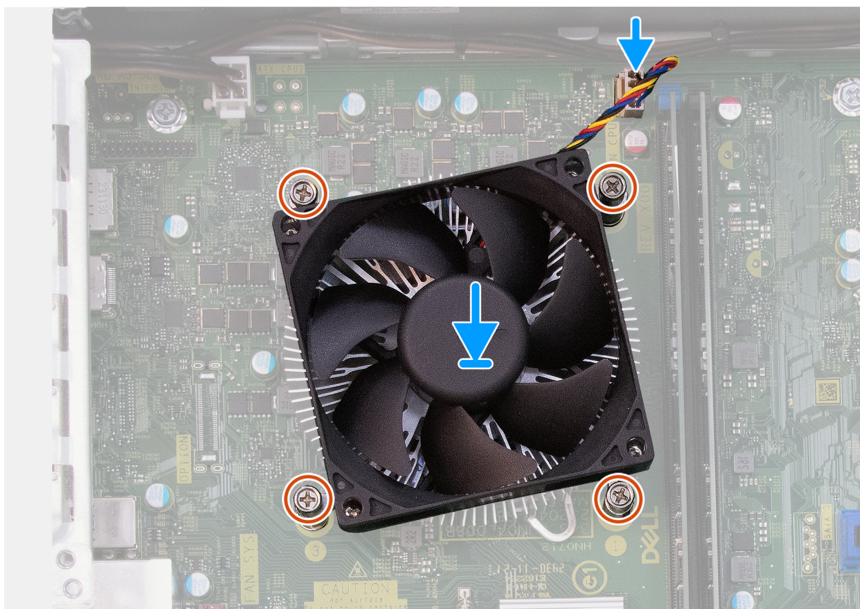
Obrázek 40. Montáž sestavy ventilátoru a chladiče procesoru
