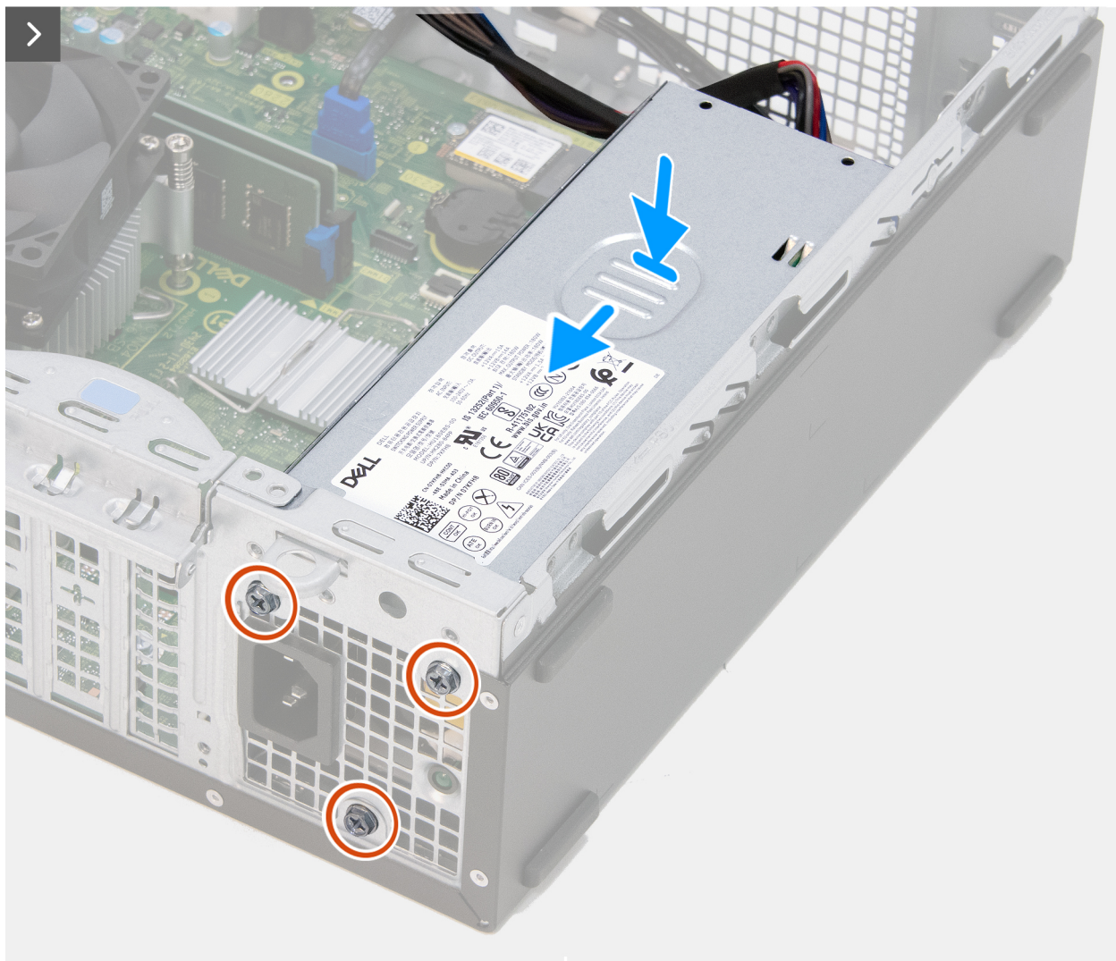
Obrázek 35. Montáž napájecího zdroje
