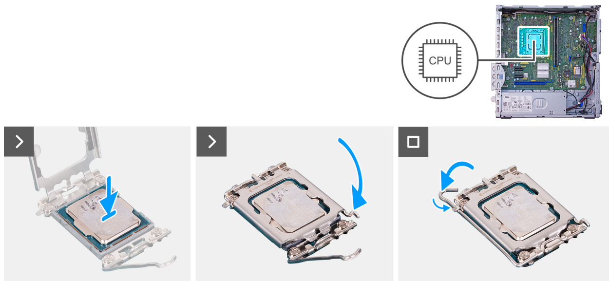
Obrázek 42. Montáž procesoru
