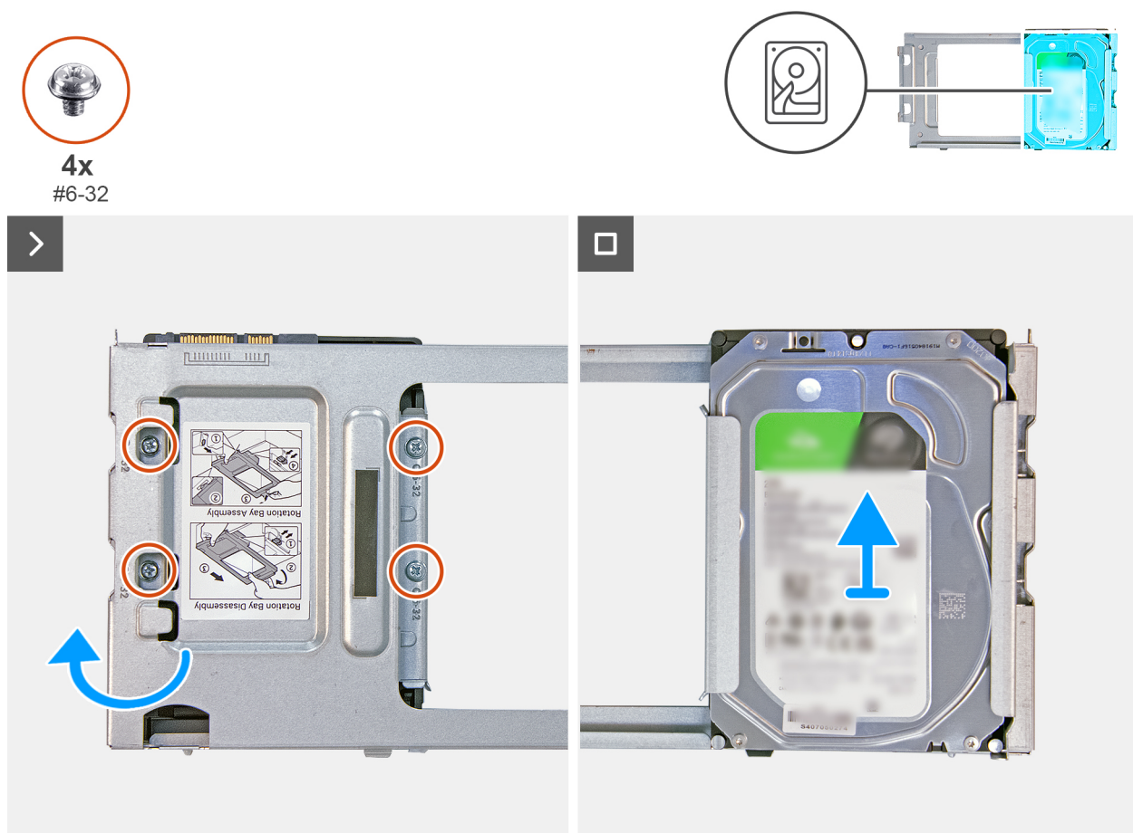
Obrázek 21. Vyjmutí pevného disku
