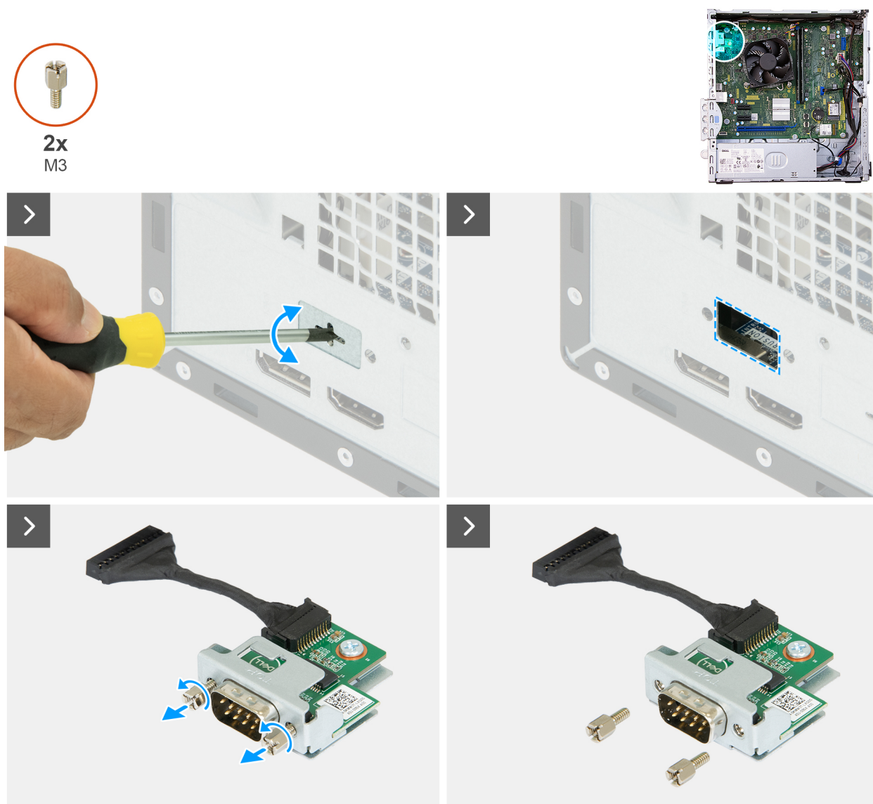
Obrázek 46. Montáž modulu sériového portu
