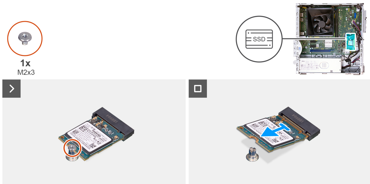
Obrázek 25. Demontáž disku SSD M.2 2230
