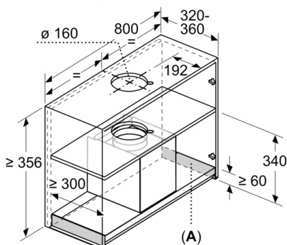
Rozměry v mm Příklad vestavby
