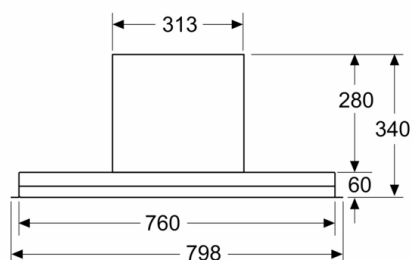
Rozměry v mm Čelní pohled
