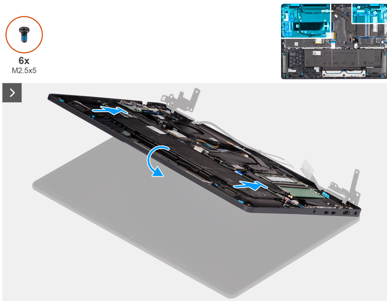
Obrázek 65. Installing the display assembly
