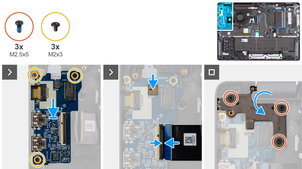
Obrázek 37. Installing the I/O board
