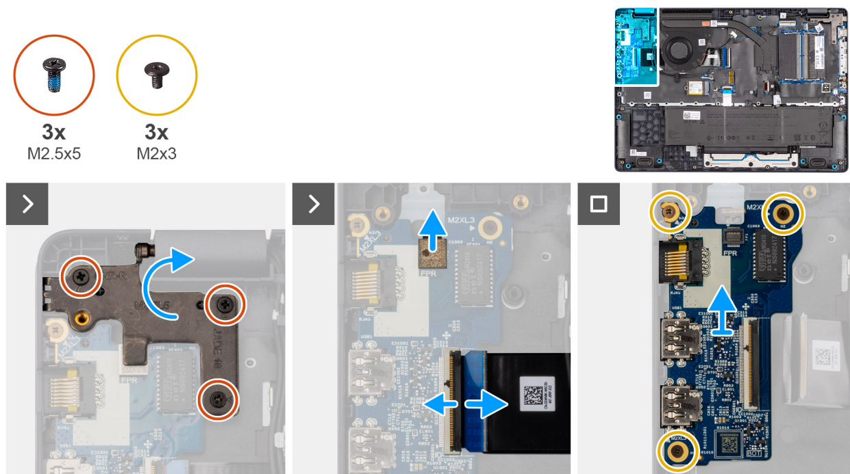
Obrázek 36. Removing the I/O board
