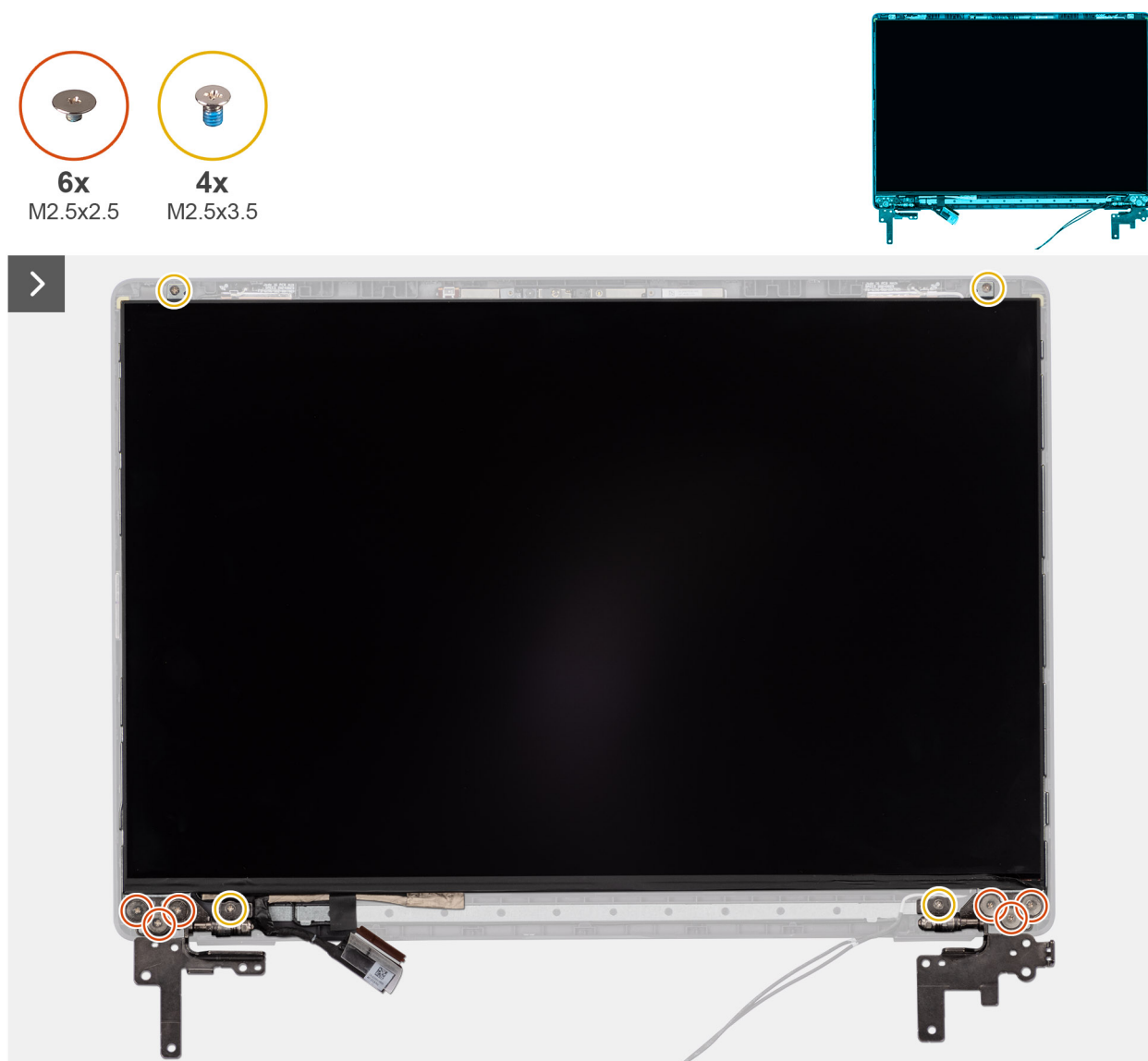
Obrázek 74. Removing the display-panel assembly
