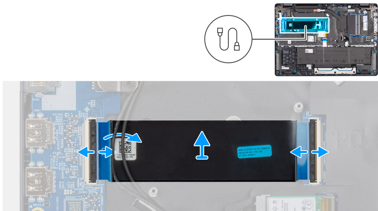
Obrázek 38. Removing the I/O-board FPC cable
