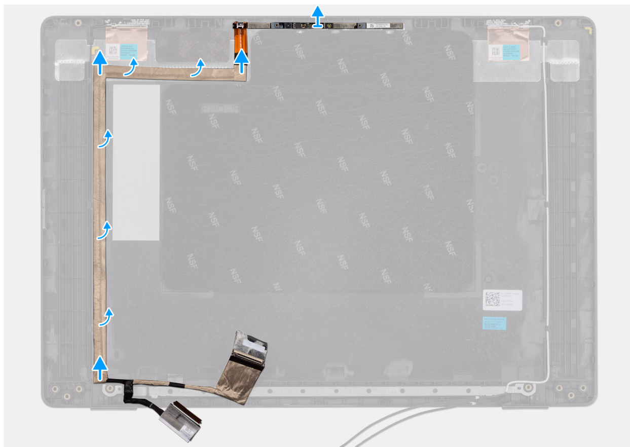
Obrázek 84. Removing the eDP cable
