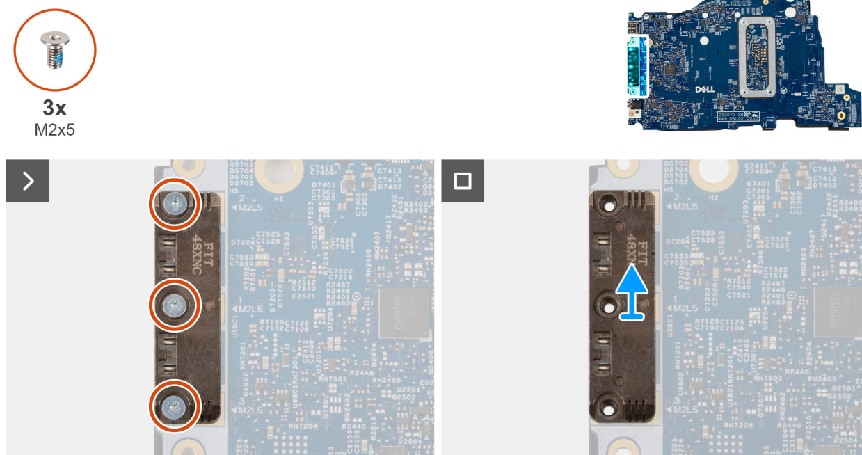
Obrázek 48. Removing the USB Type-C module
