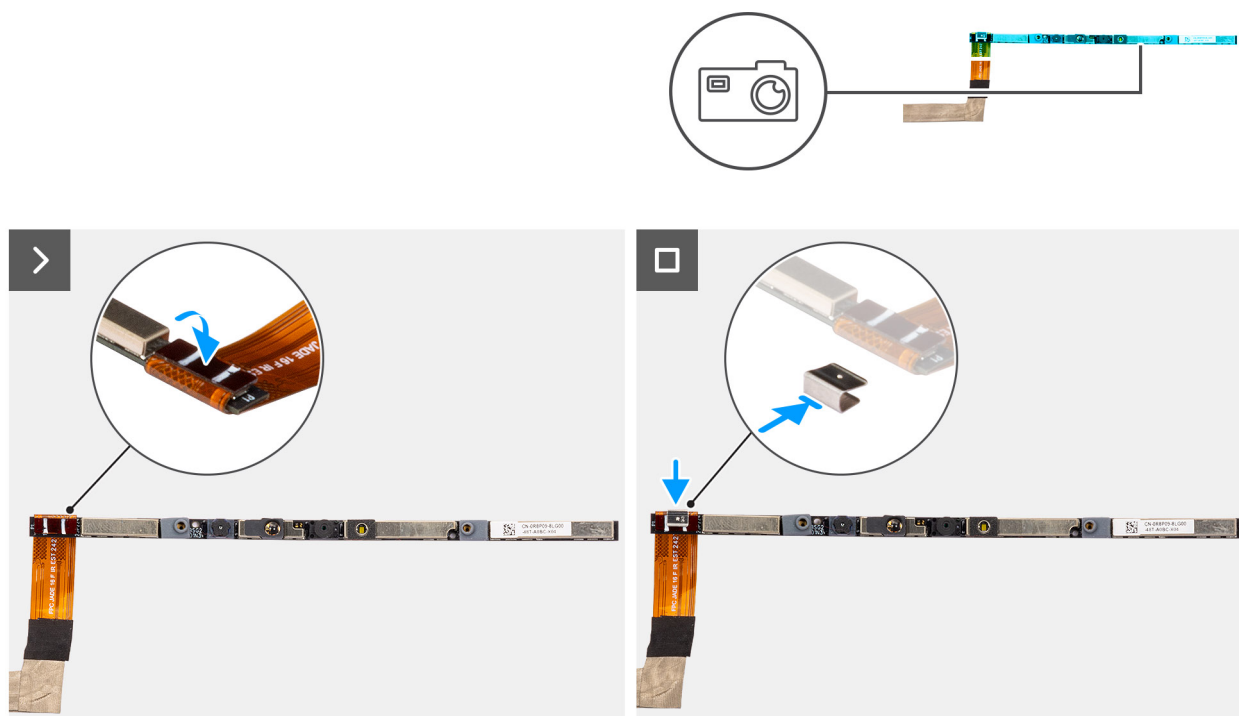
Obrázek 83. Installing the camera
