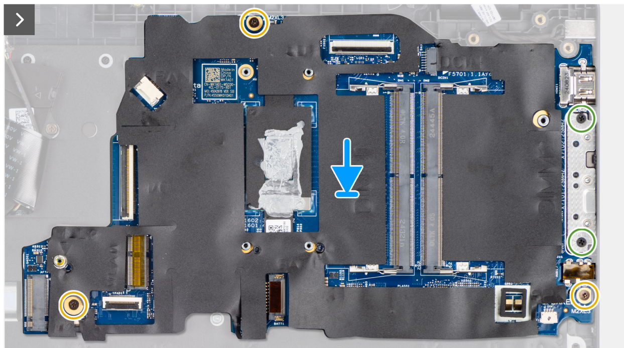
Obrázek 46. Installing the system board
