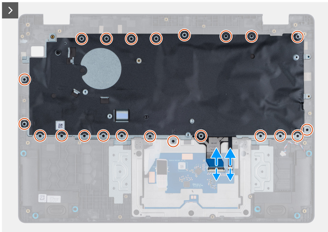
Obrázek 50. Removing the keyboard
