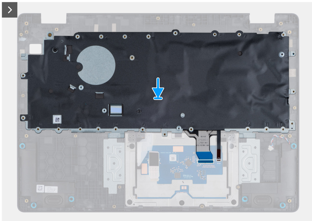
Obrázek 54. Installing the keyboard
