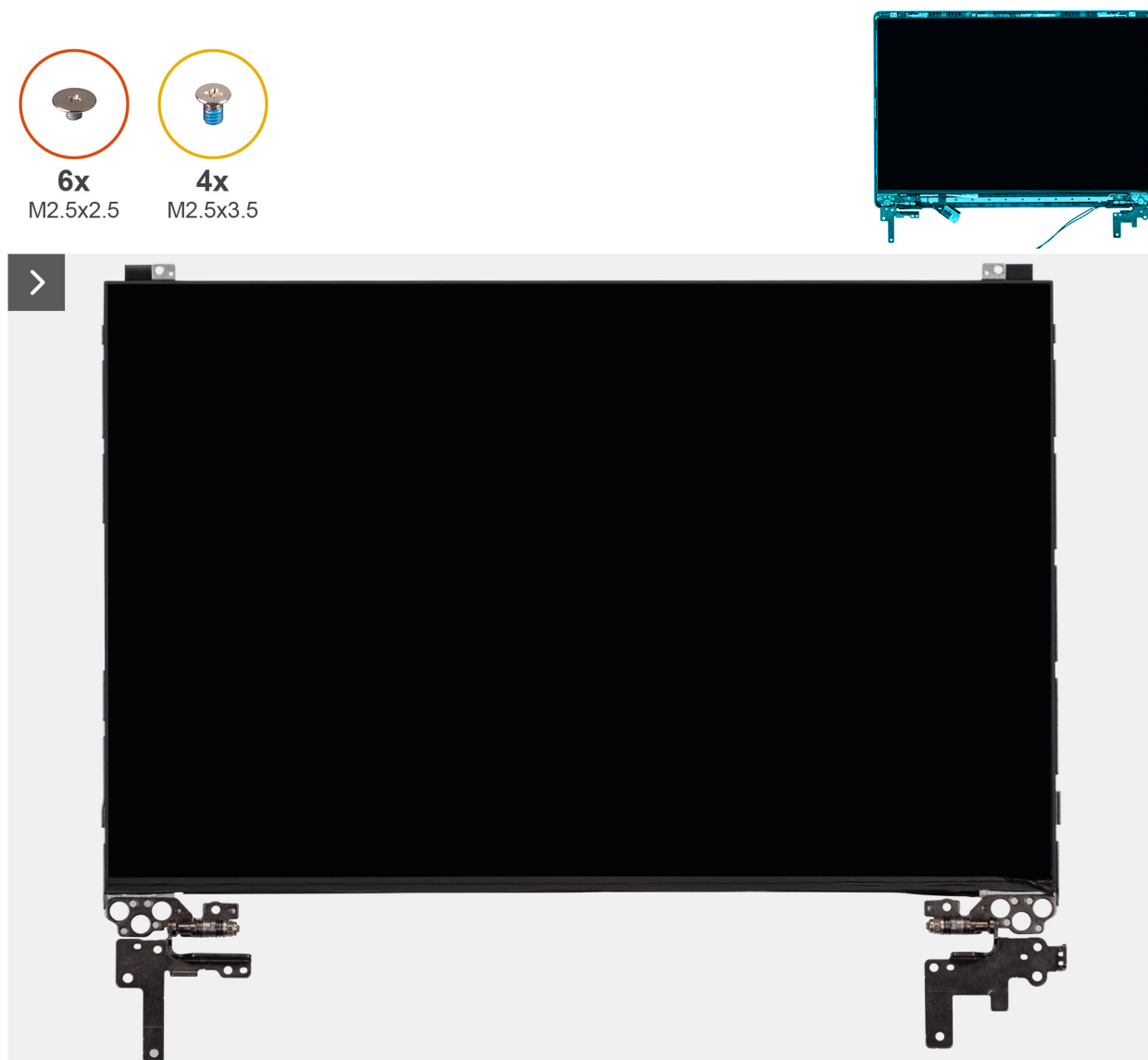
Obrázek 78. Installing the display-panel assembly
