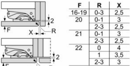
Rozměry v mm Doporučené rozměry mezer pro plochý závěs
