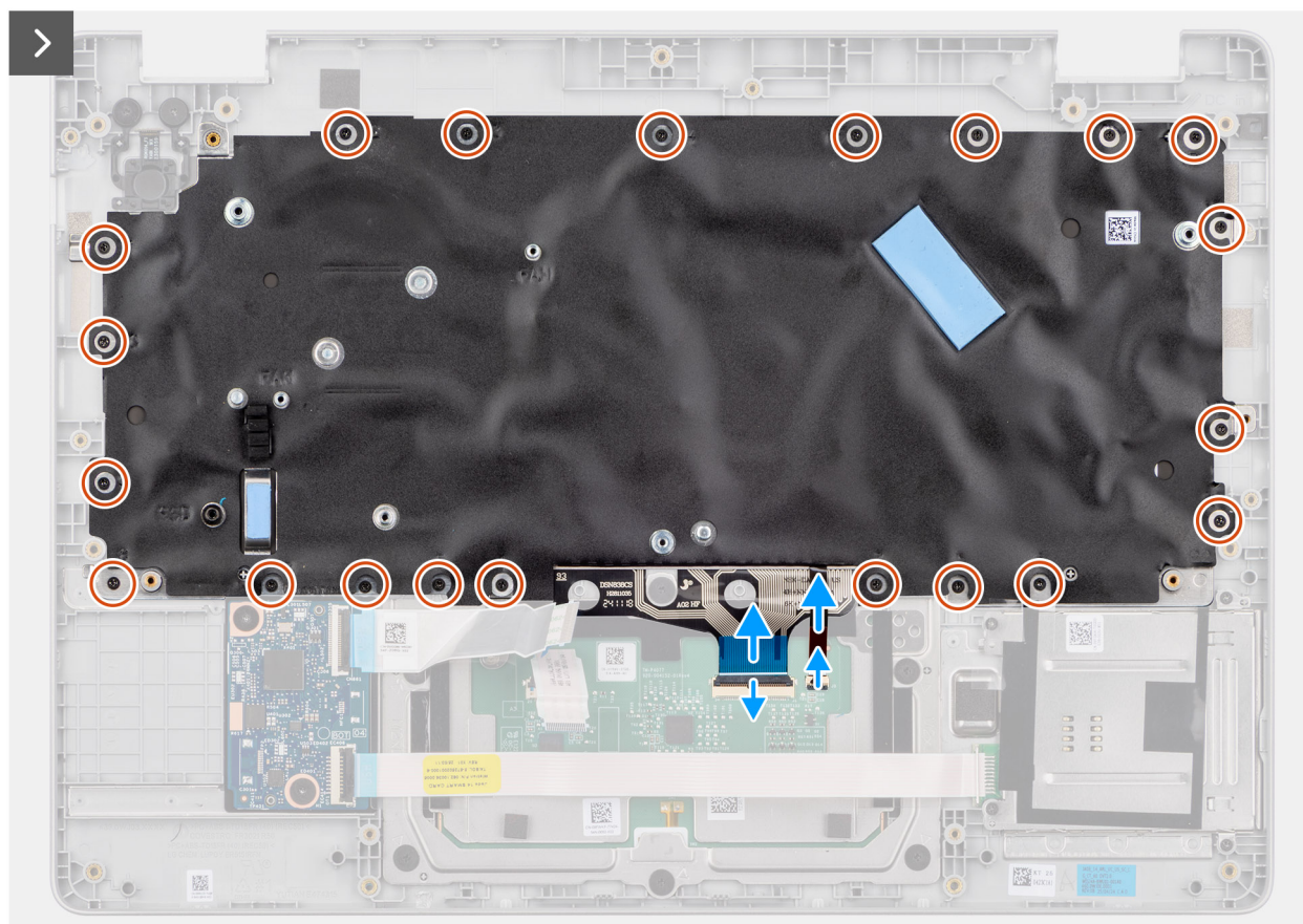
Obrázek 85. Demontáž klávesnice
