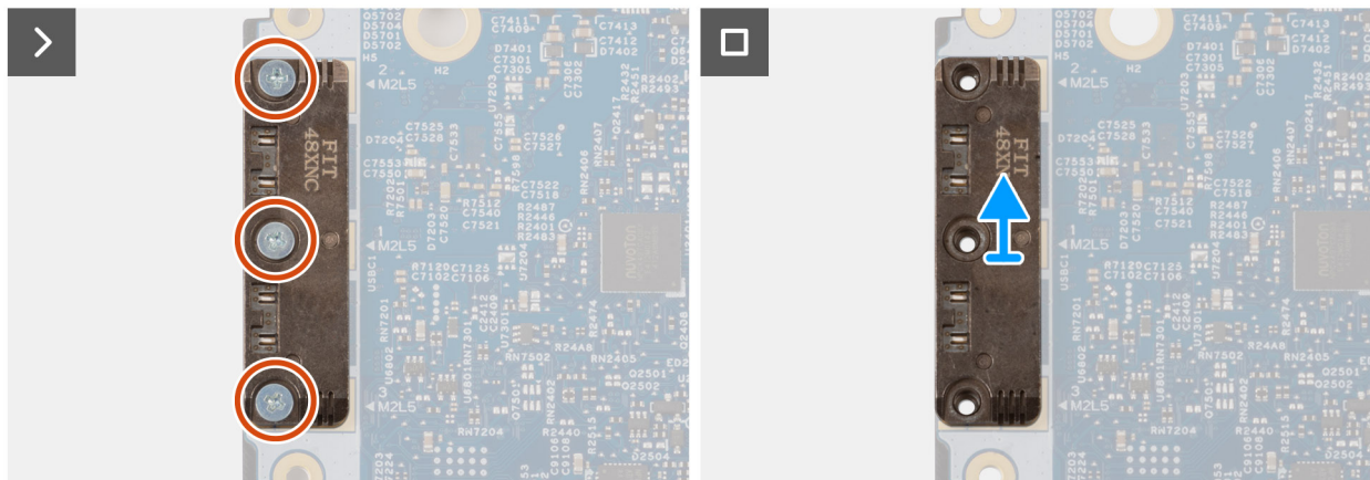
Obrázek 77. Demontáž modulu USB Type-C
