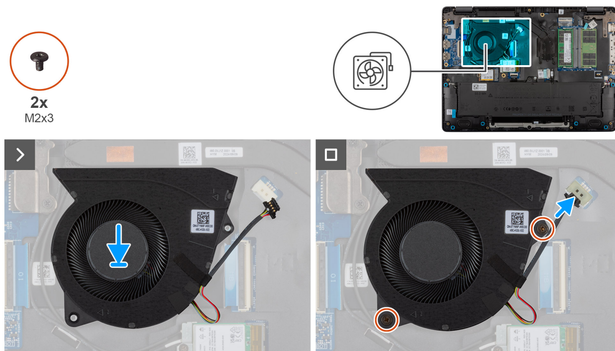
Obrázek 34. Montáž ventilátoru
