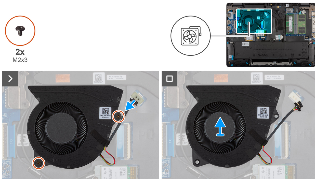
Obrázek 33. Demontáž ventilátoru
