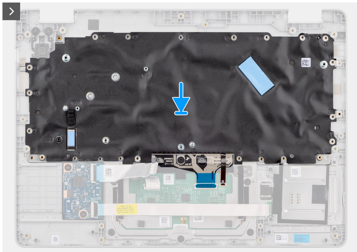
Obrázek 89. Montáž klávesnice
