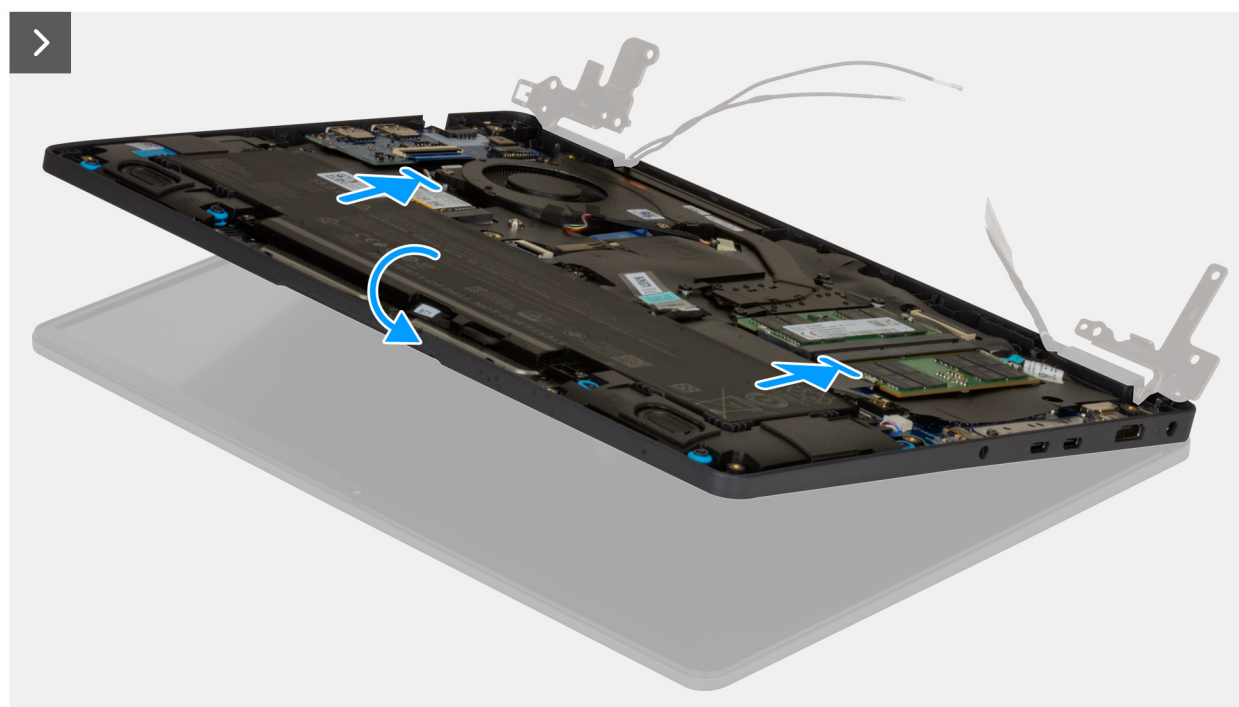
Obrázek 102. Montáž sestavy displeje
