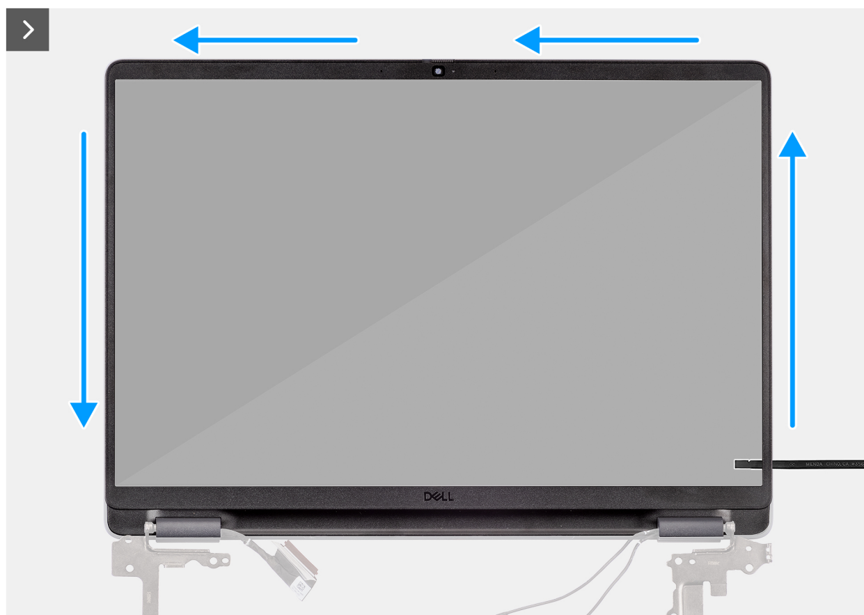
Obrázek 107. Demontáž čelního krytu displeje
