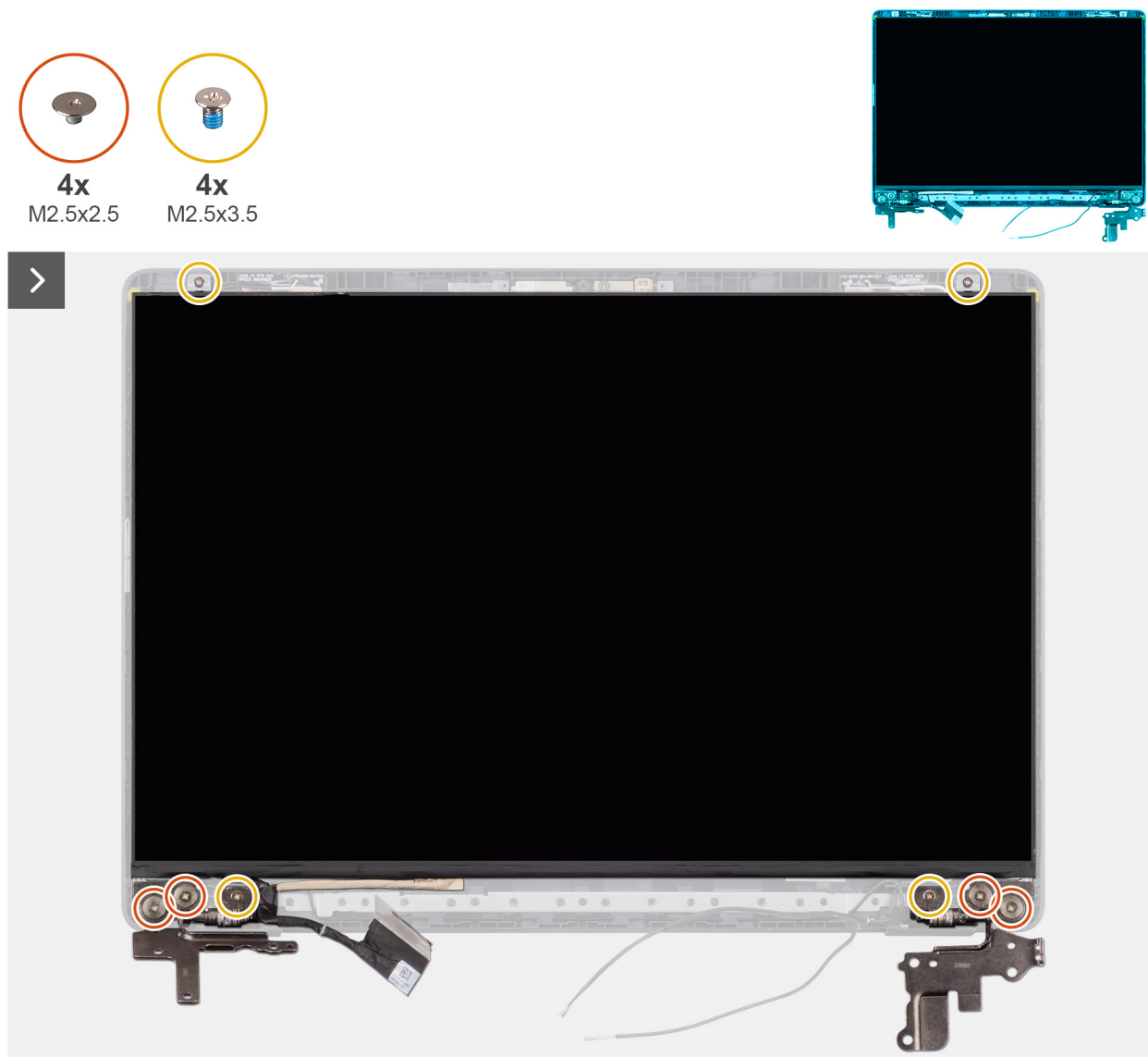
Obrázek 111. Demontáž sestavy obrazovky displeje
