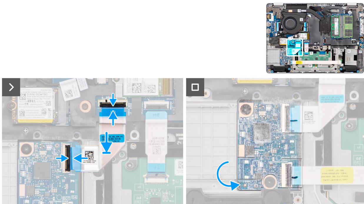
Obrázek 36. Montáž plochého kabelu desky USH
