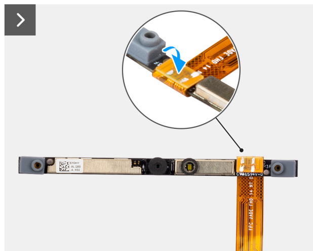
Obrázek 120. Montáž kamery
