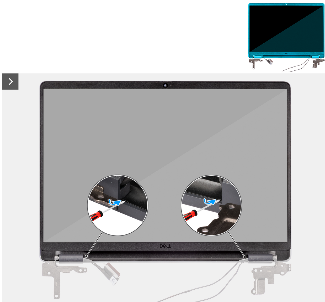
Obrázek 104. Demontáž čelního krytu displeje
