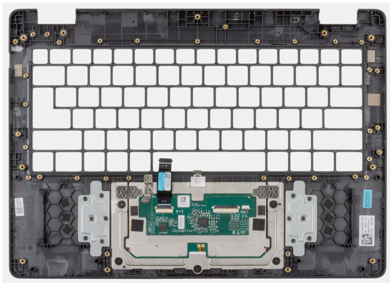
Obrázek 96. Montáž sestavy opěrky pro dlaň
