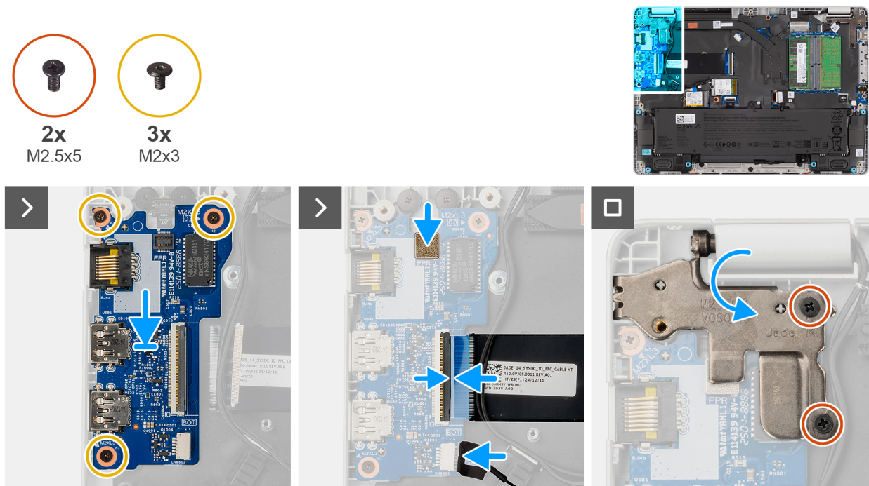
Obrázek 52. Vložení desky I/O
