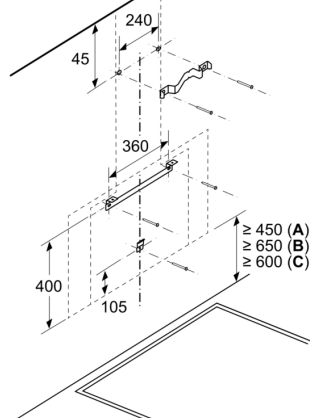
Rozměry v mm Nástěnná instalace s komínem
