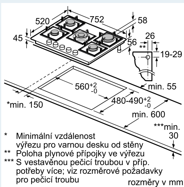
Rozměrové výkresy
