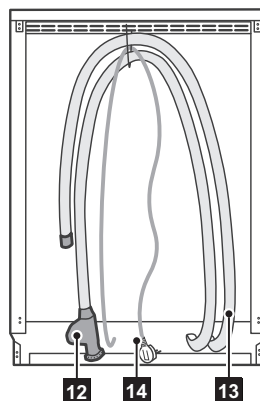
Pohľad zozadu
