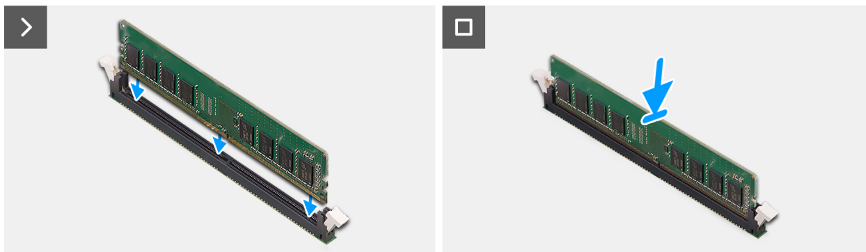
Obrázek 23. Vložení paměťového modulu
