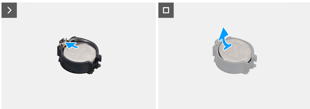
Obrázek 14. Vyjmutí knoflíkové baterie
