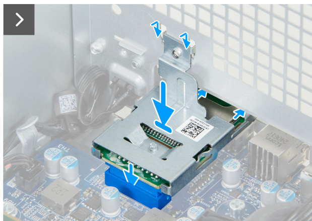
Obrázek 29. Montáž čtečky paměťových karet
