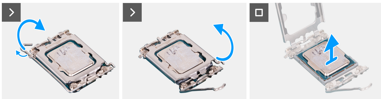
Obrázek 40. Demontáž procesoru
