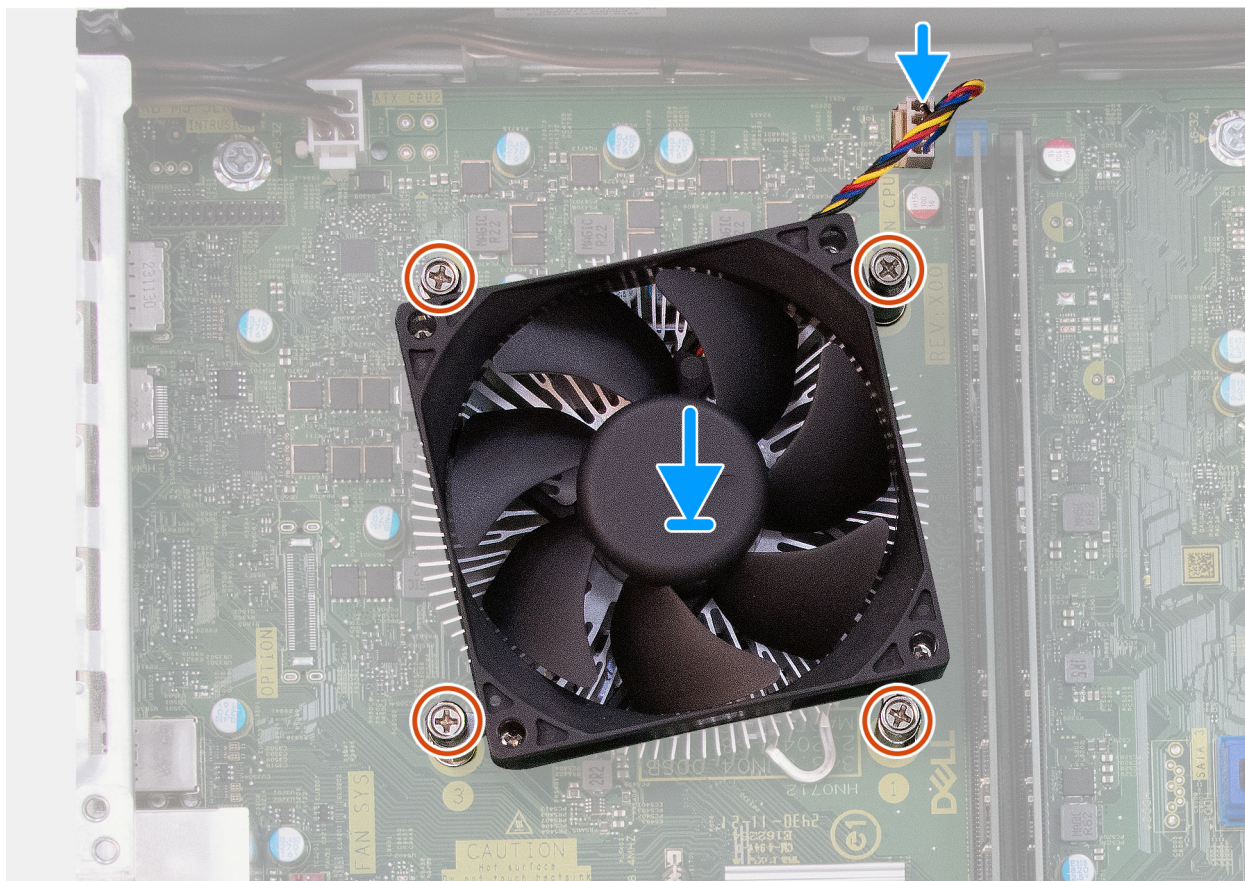
Obrázek 39. Montáž sestavy ventilátoru a chladiče procesoru
