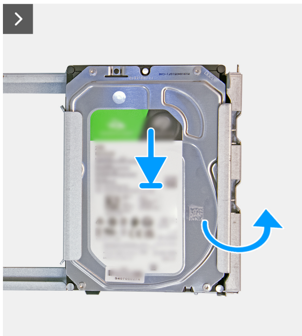
Obrázek 21. Montáž pevného disku
