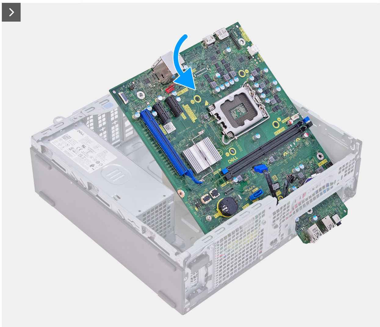
Obrázek 52. Montáž základní desky
