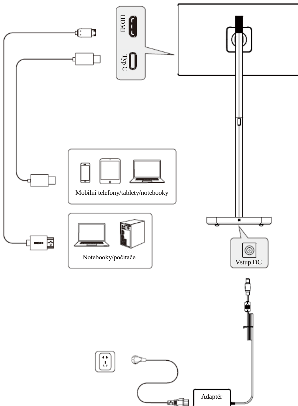
Obrázek 4-1 Vstupní a výstupní rozhraní
