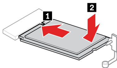
Obrázek 7. Nainstalujte novou jednotku SSD M.2
