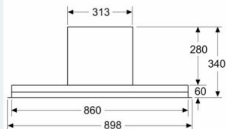
Rozměry v mm Čelní pohled
