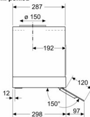
Rozměry v mm Boční pohled
