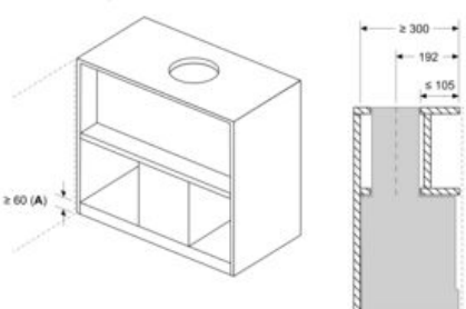
Rozměry v mm Příklad instalace s políci na koření
