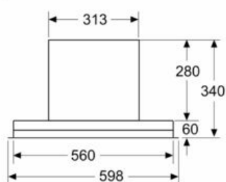
Rozměry v mm Čelní pohled
