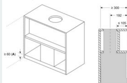
Rozměry v mm Příklad instalace s polici na kořeni
