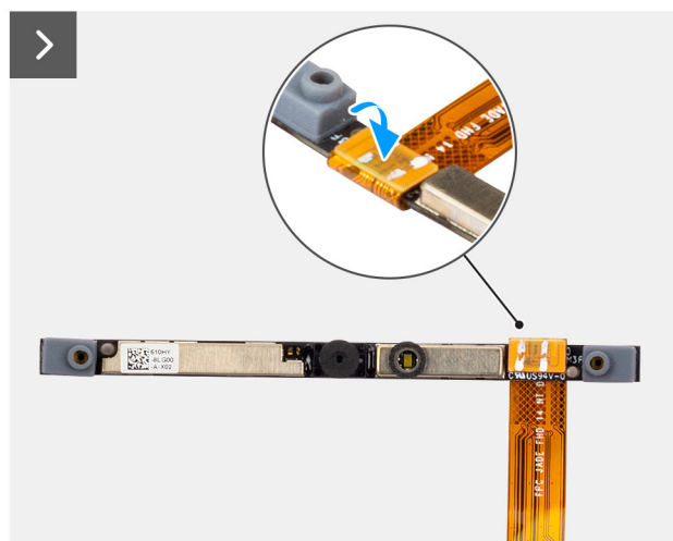
Obrázek 83. Montáž kamery
