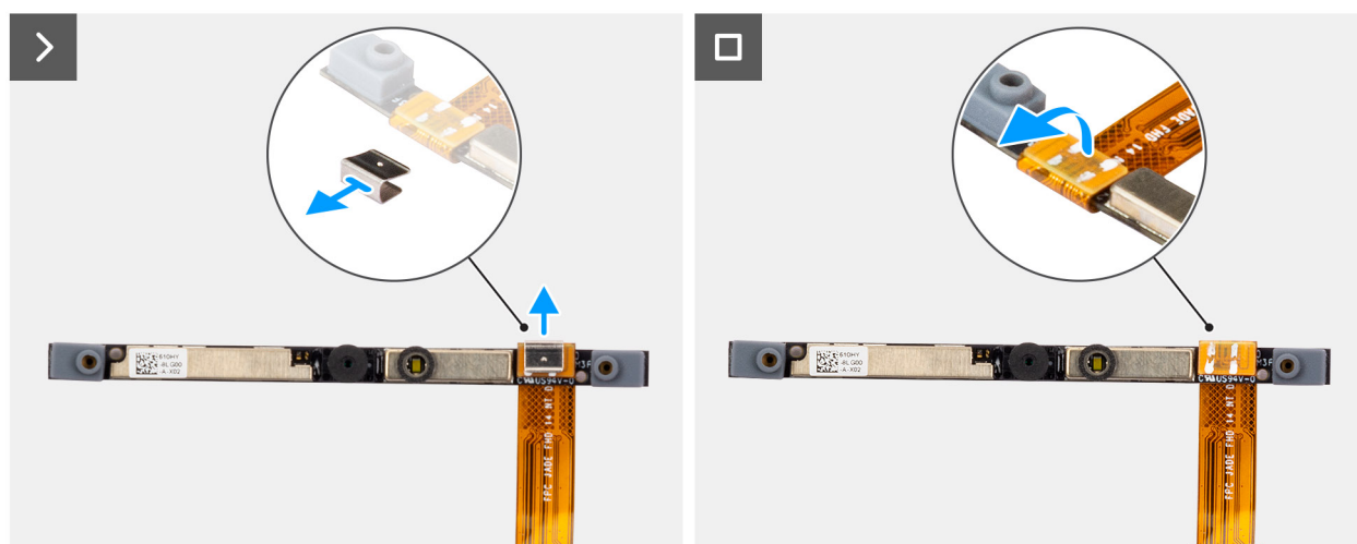
Obrázek 82. Demontáž kamery
