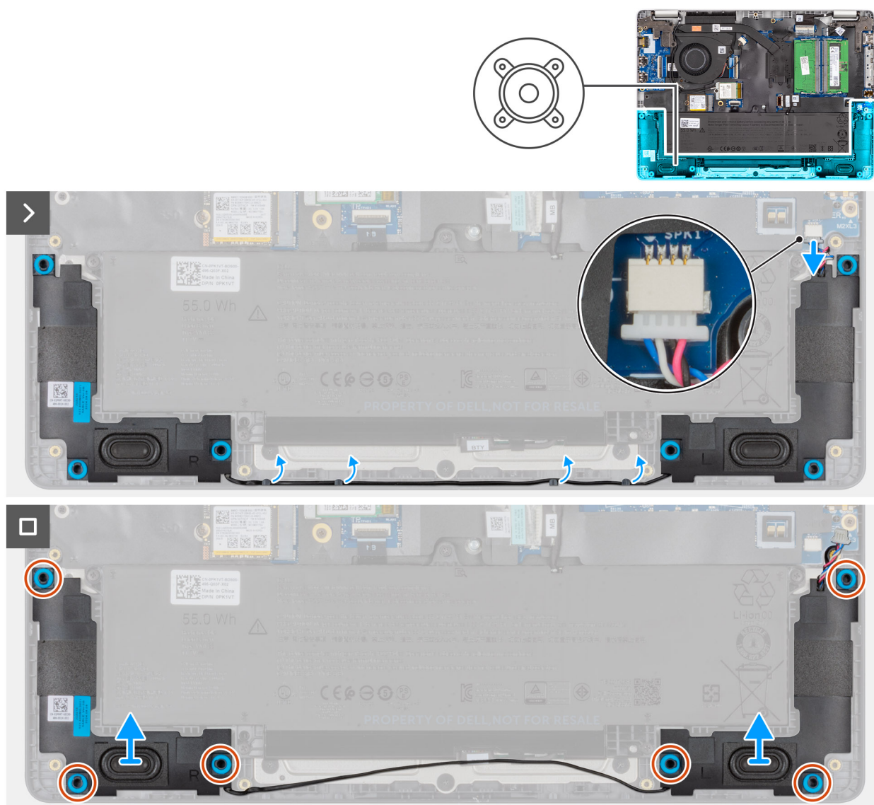
Obrázek 27. Demontáž reproduktorů
