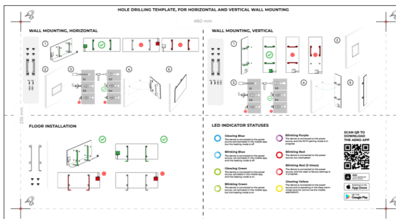
Šablona pro vrtání otvorů do stěny
