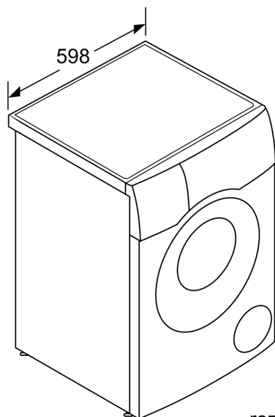
Rozměrové výkresy
