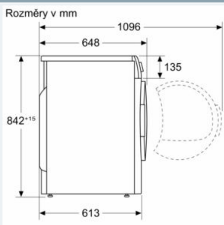
Rozměrové výkresy
