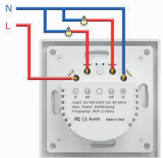
SCHÉMA ZAPOJENÍ
