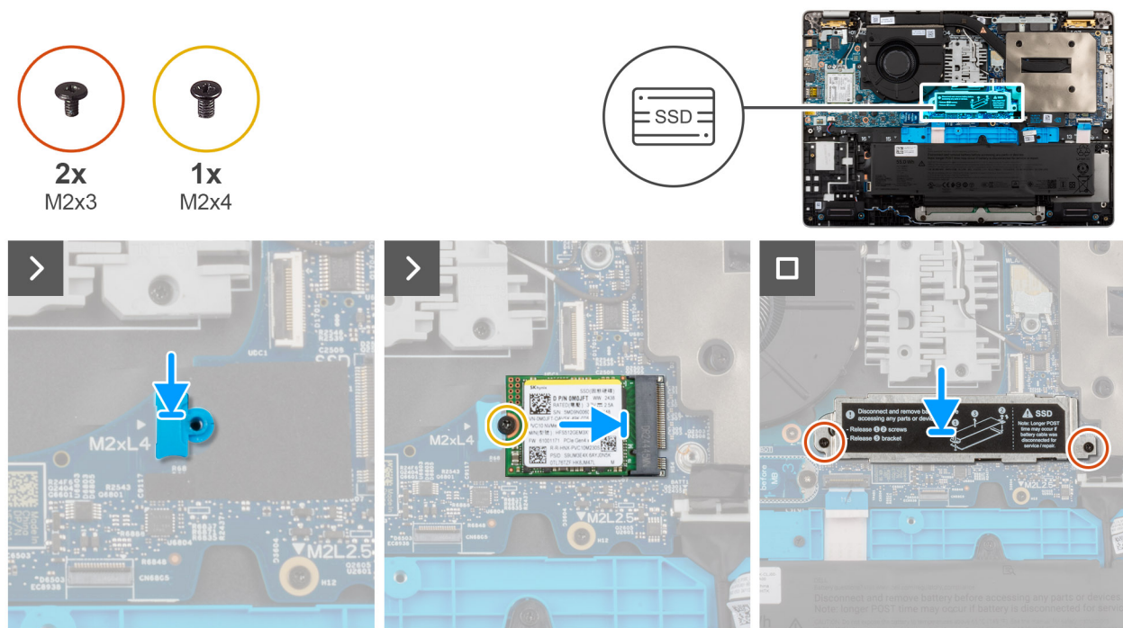
Obrázek 25. Montáž disku SSD M.2 2230
