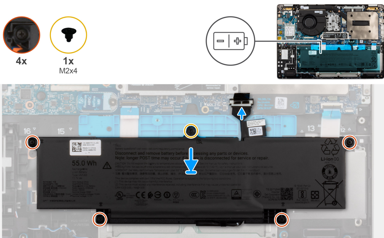
Obrázek 20. Vložení baterie
