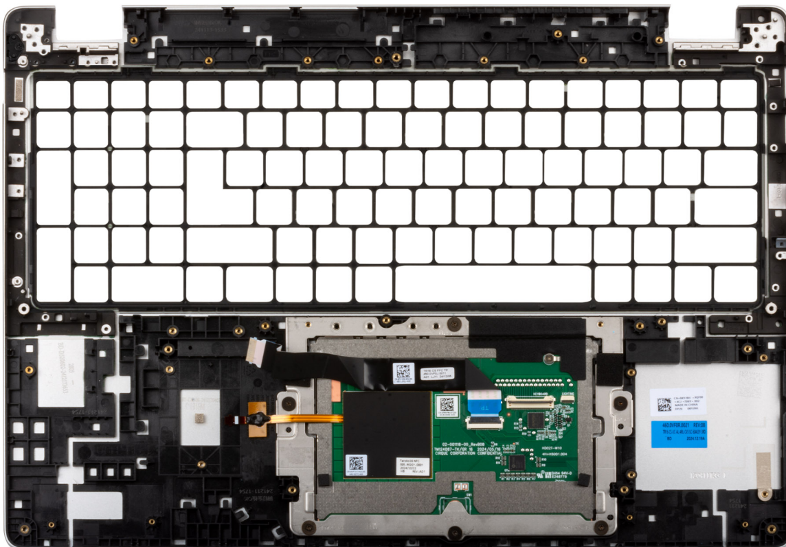
Obrázek 83. Demontáž sestavy opěrky pro dlaň
