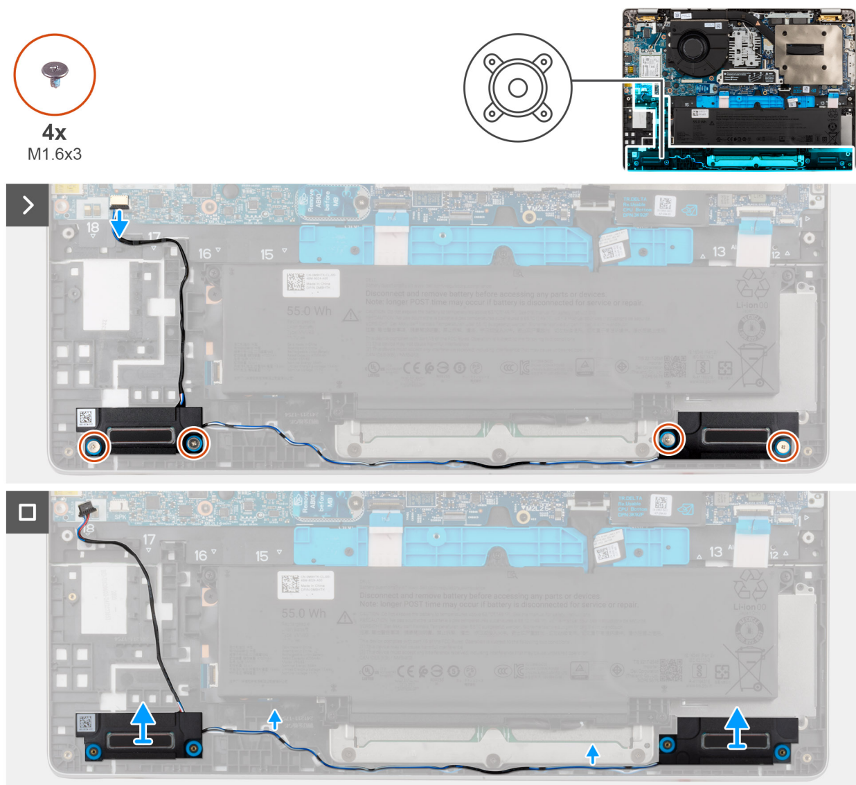
Obrázek 30. Demontáž reproduktorů
