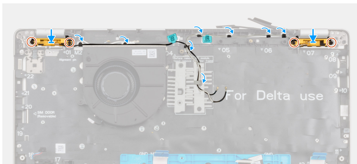
Obrázek 77. Montáž bezdrátové antény
