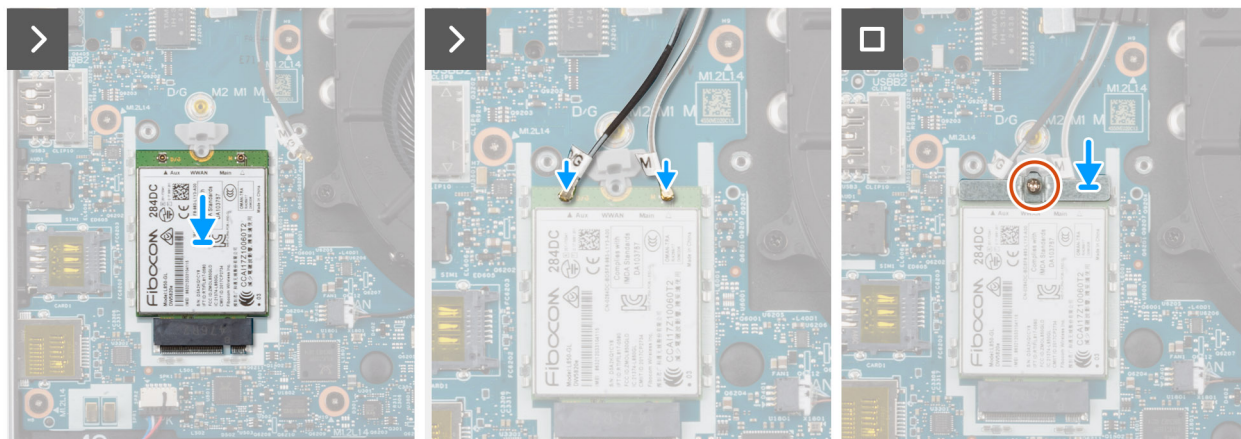
Obrázek 29. Montáž karty 4G WWAN
