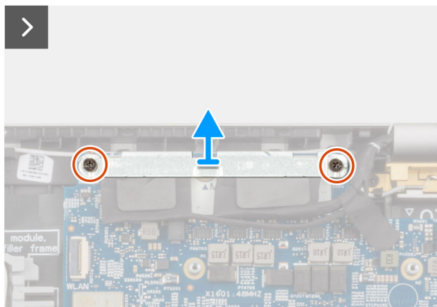
Obrázek 52. Demontáž sestavy displeje
