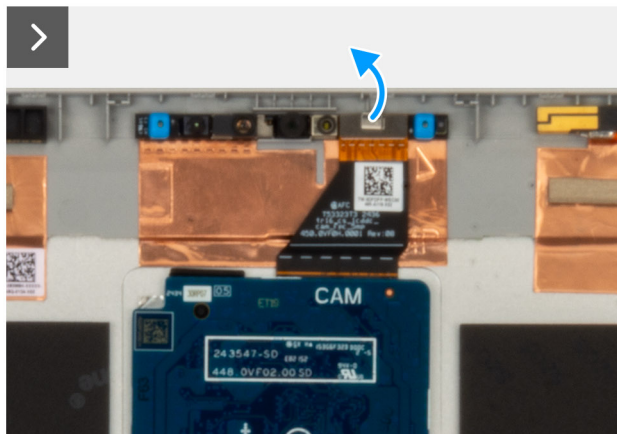
Obrázek 72. Demontáž modulu kamery
