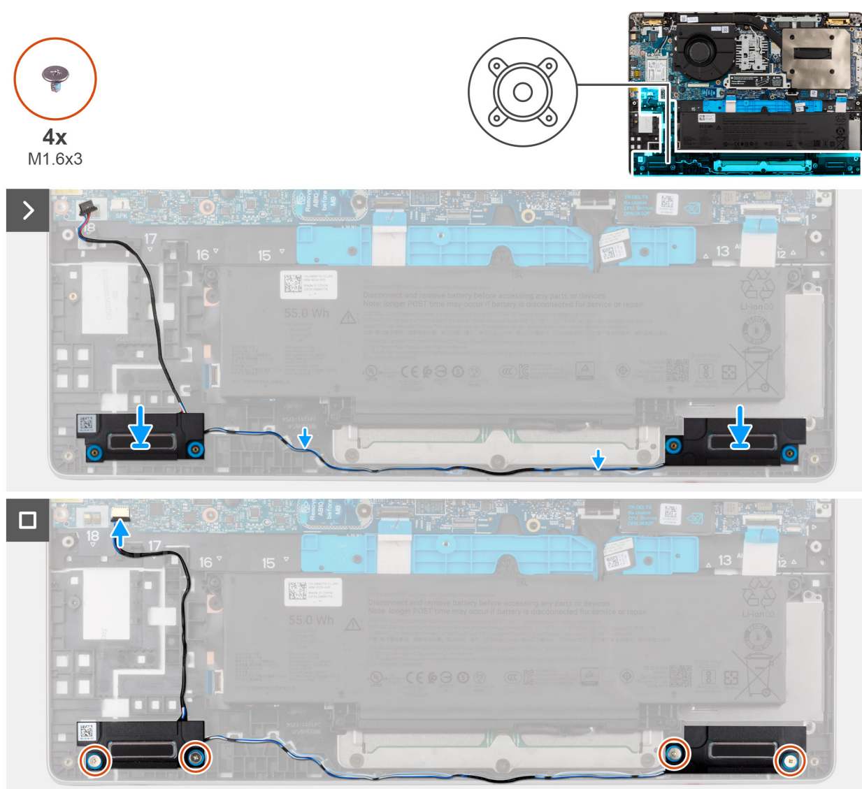
Obrázek 31. Montáž reproduktorů
