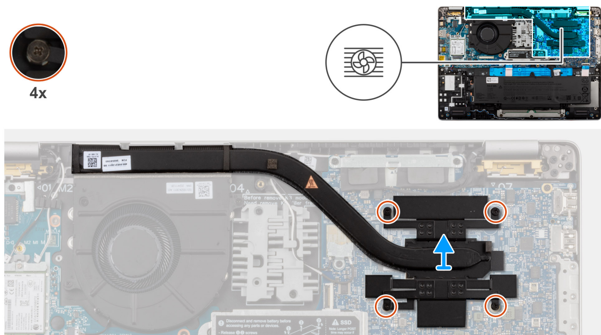
Obrázek 40. Demontáž chladiče
