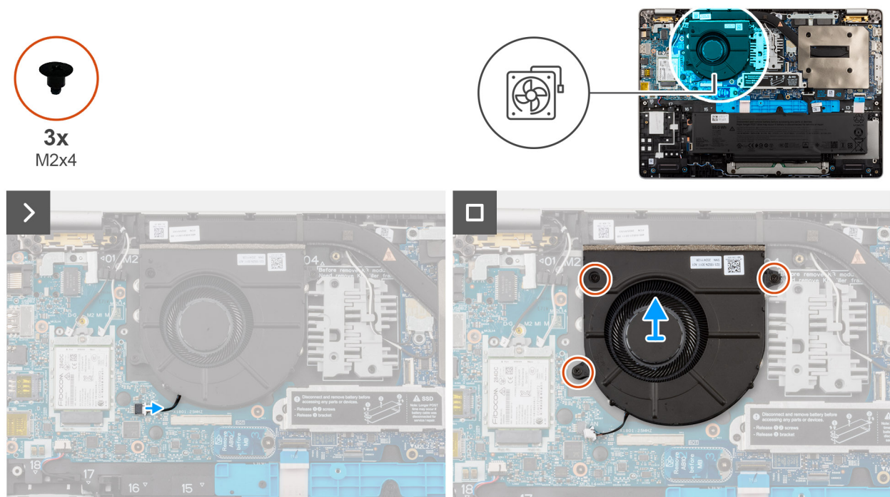
Obrázek 32. Demontáž ventilátoru
