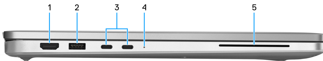
Obrázek 2. Pohled zleva
