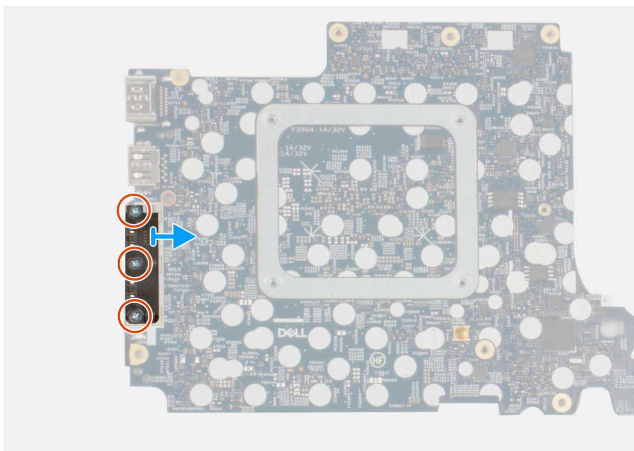
Obrázek 48. Demontáž modulu konektoru USB Type-C
