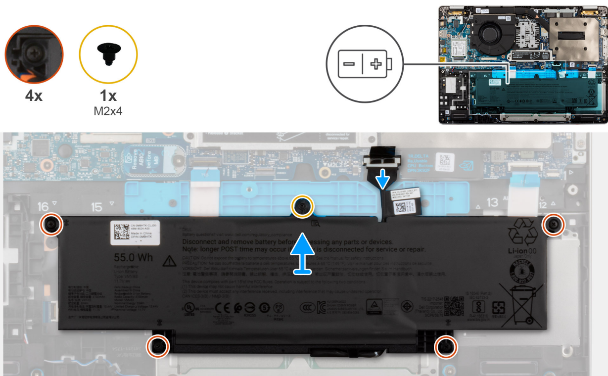
Obrázek 19. Vyjmutí baterie
