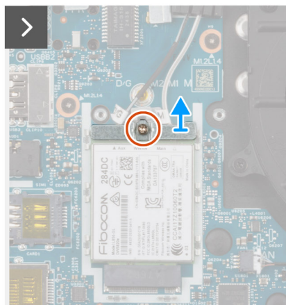
Obrázek 28. Vyjmutí karty 4G WWAN
