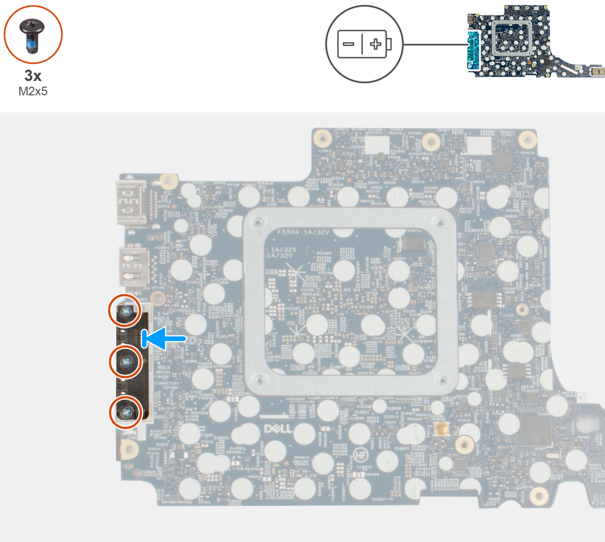
Obrázek 49. Montáž modulu konektoru USB Type-C
