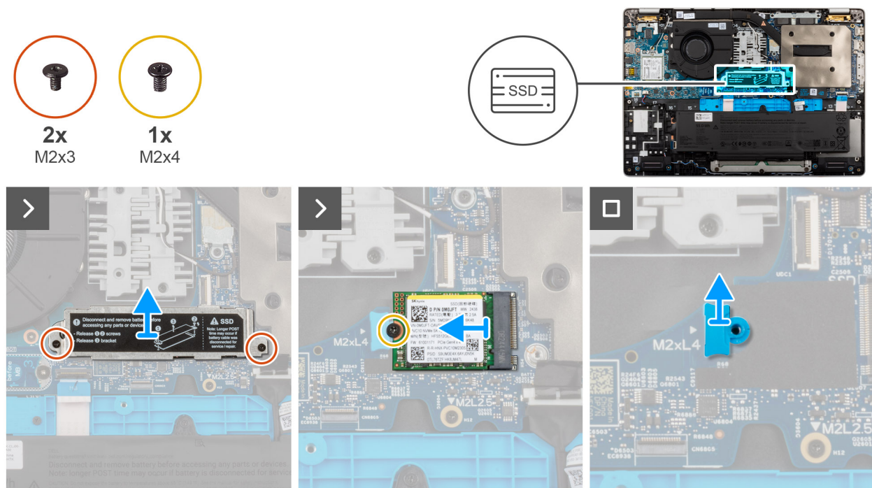
Obrázek 24. Demontáž disku SSD M.2 2230
