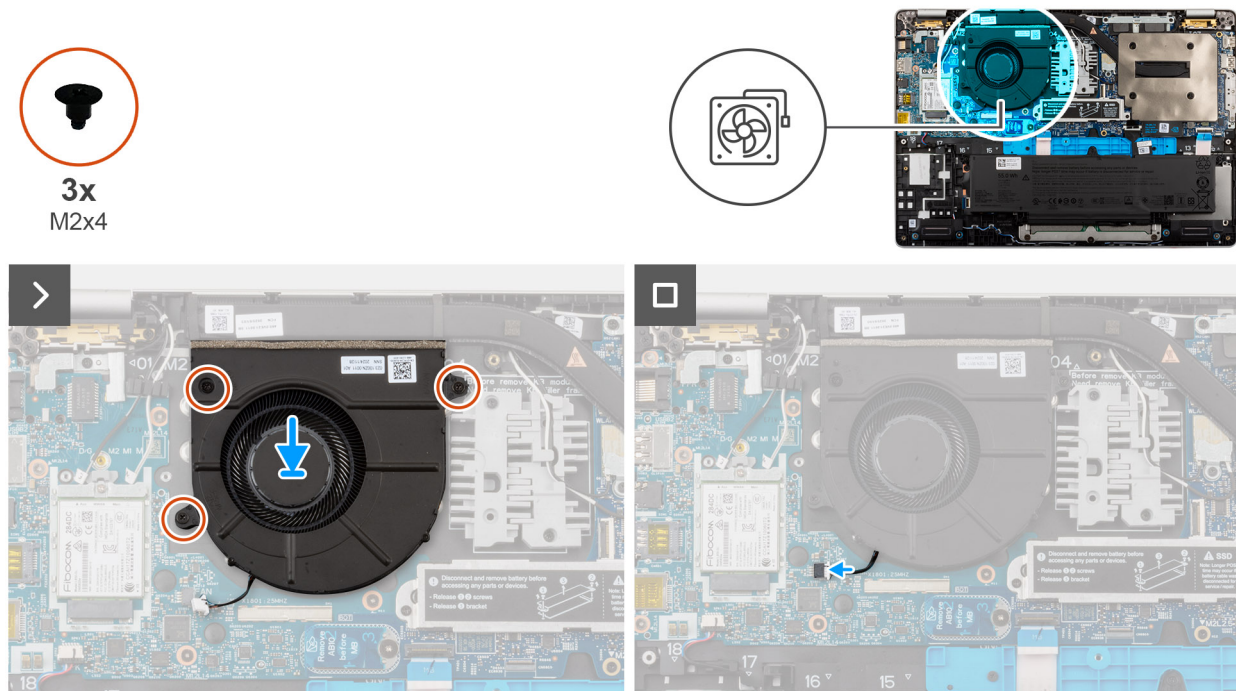
Obrázek 33. Montáž ventilátoru
