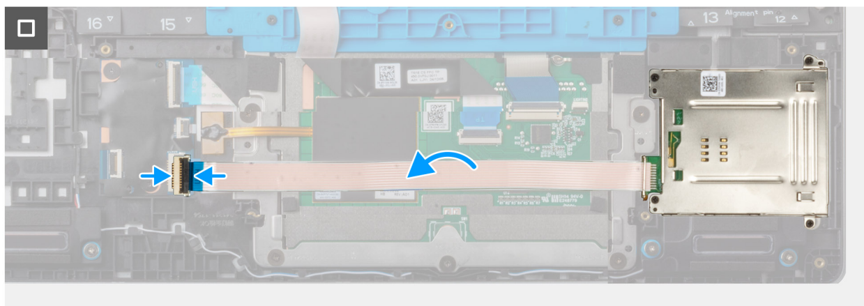
Obrázek 37. Montáž čtečky čipových karet
