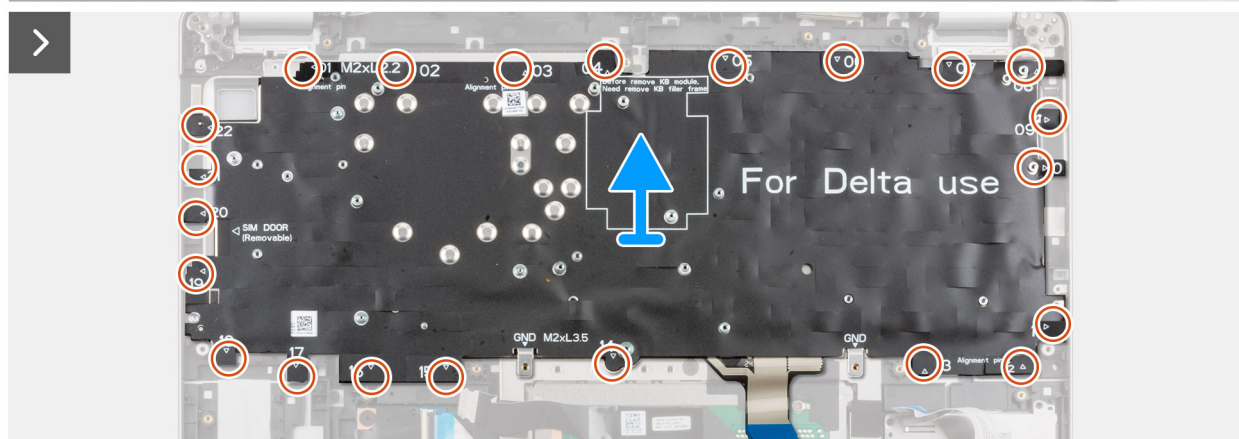
Obrázek 78. Demontáž klávesnice
