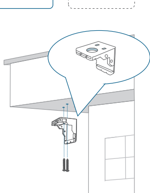
Stropní montáž
