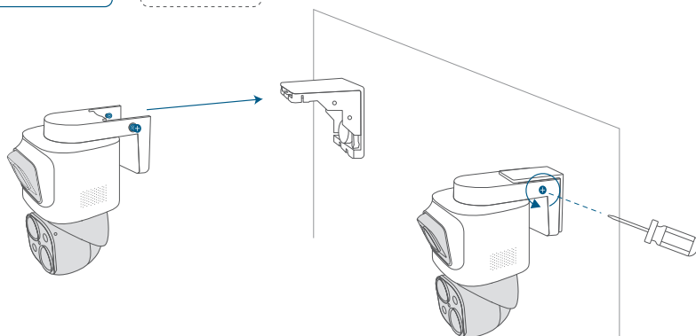
① Vložte kameru
