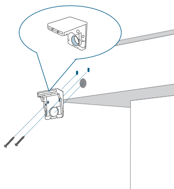
Montáž na stěnu
