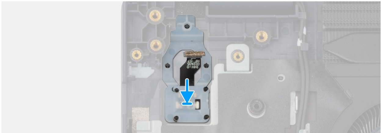
Obrázek 41. Montáž vypínače se čtečkou otisků prstů
