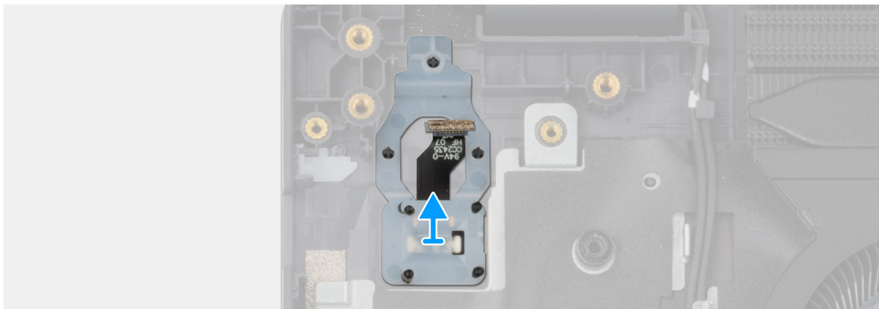
Obrázek 40. Demontáž vypínače se čtečkou otisků prstů
