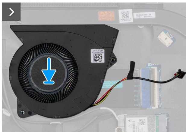
Obrázek 31. Montáž ventilátoru
