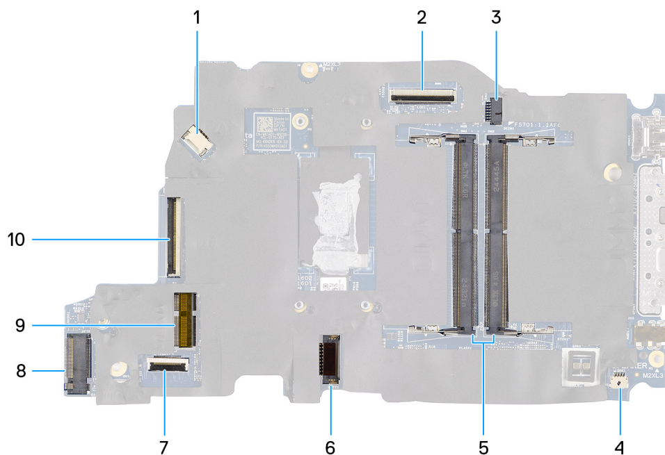
Obrázek 45. Konektory na základní desce
