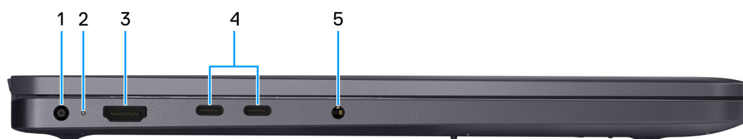
Obrázek 2. Pohled zleva
