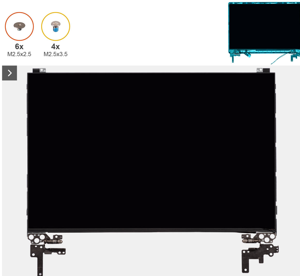
Obrázek 78. Montáž sestavy obrazovky displeje
