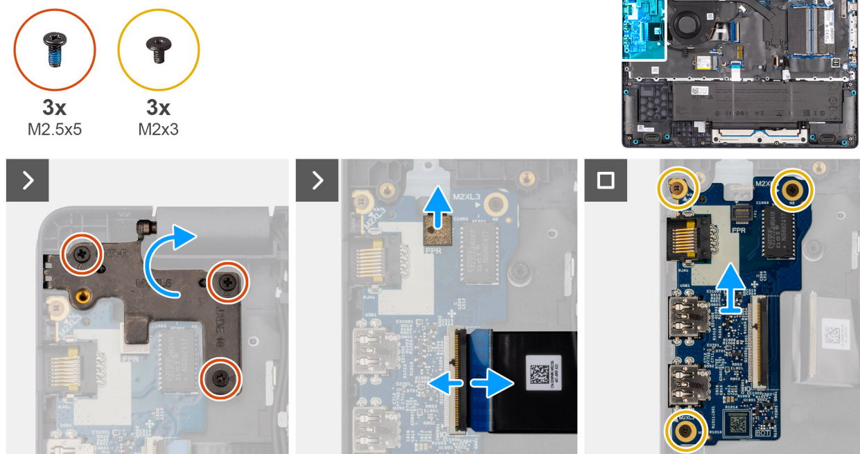
Obrázek 36. Demontáž desky I/O
