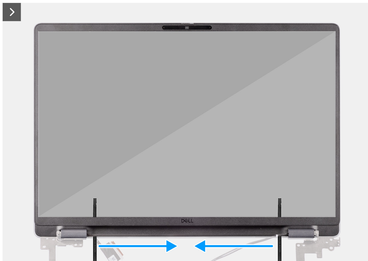
Obrázek 68. Demontáž čelního krytu displeje
