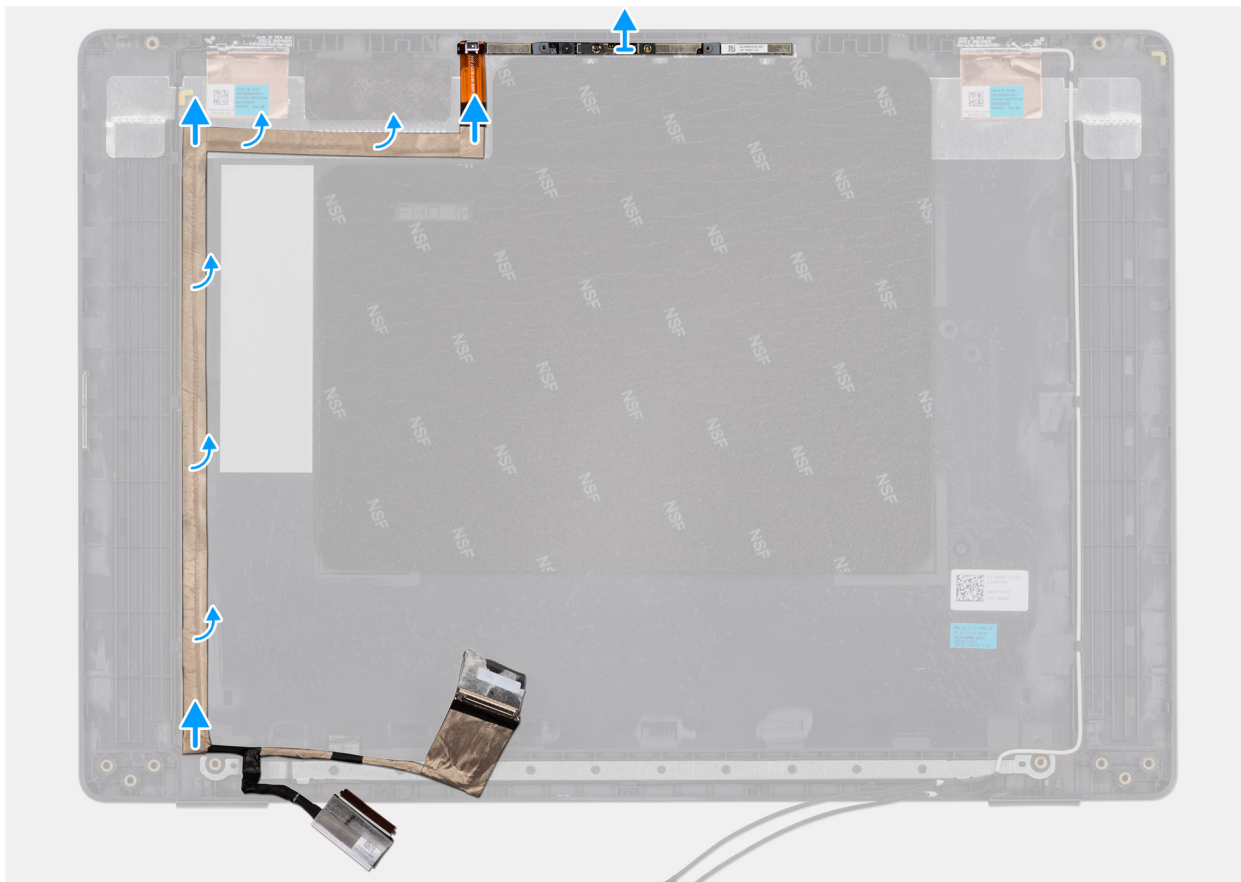
Obrázek 84. Vyjmutí kabelu eDP
