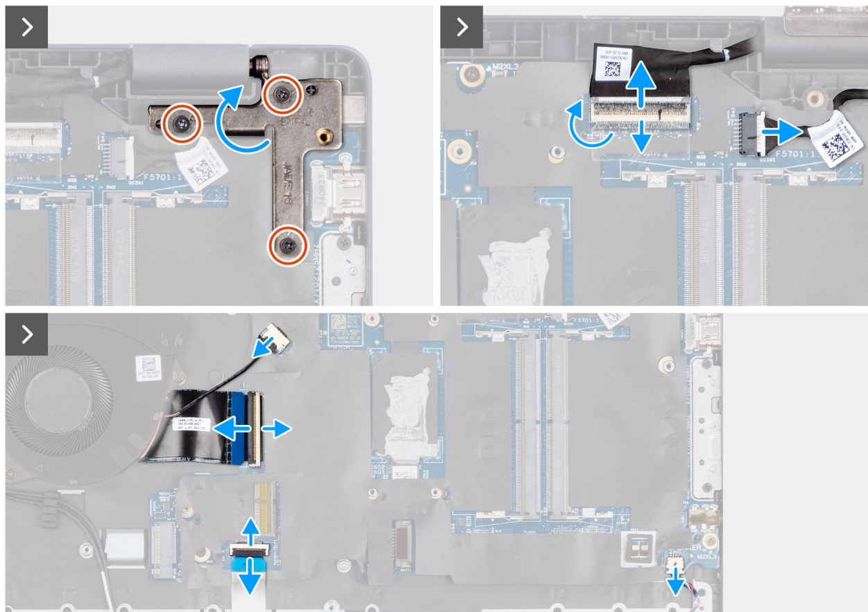
Obrázek 43. Demontáž základní desky
