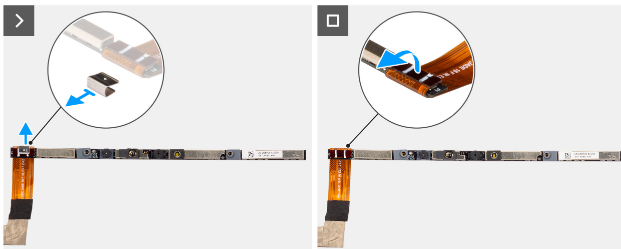
Obrázek 82. Demontáž kamery
