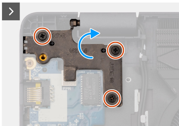
Obrázek 62. Demontáž sestavy displeje
