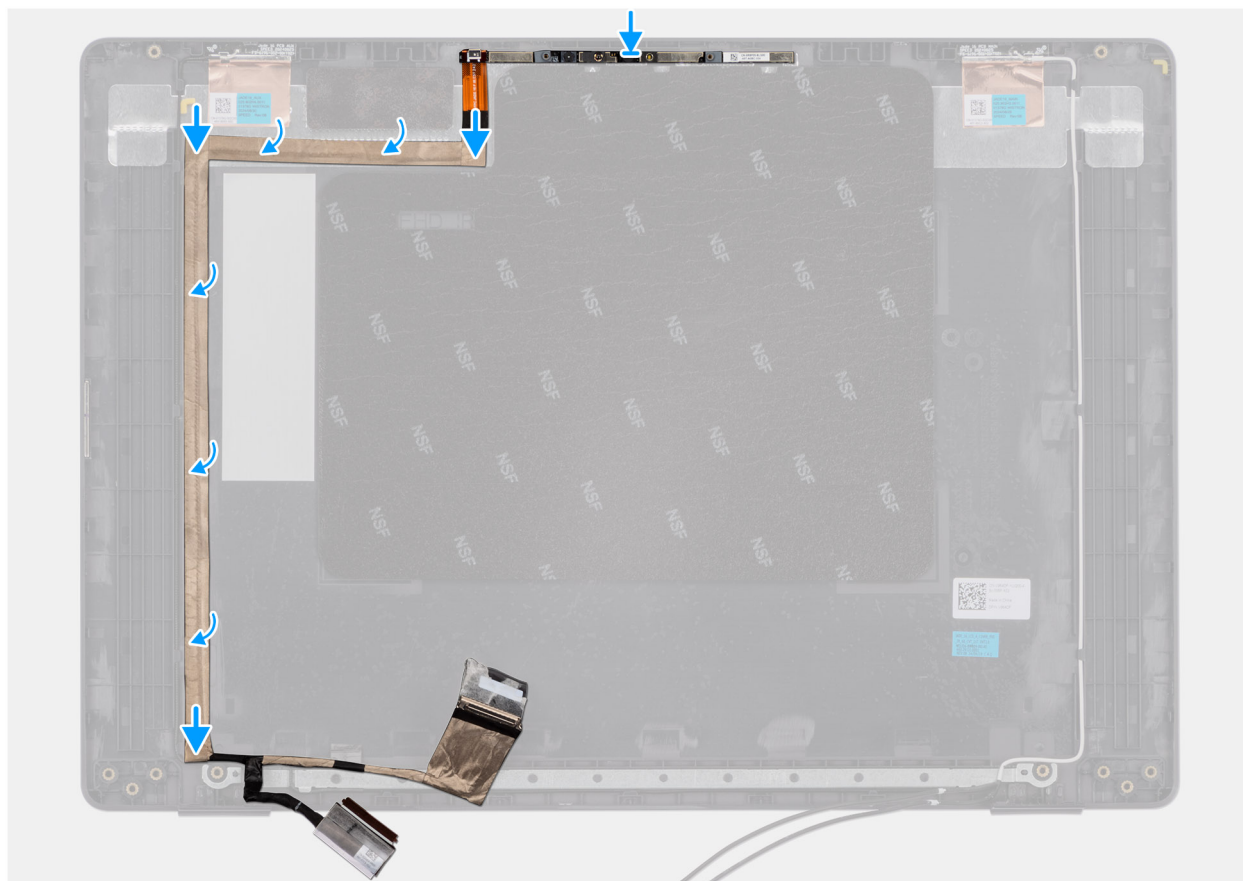
Obrázek 85. Montáž kabelu eDP
