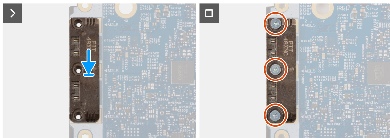
Obrázek 49. Montáž modulu USB Type-C
