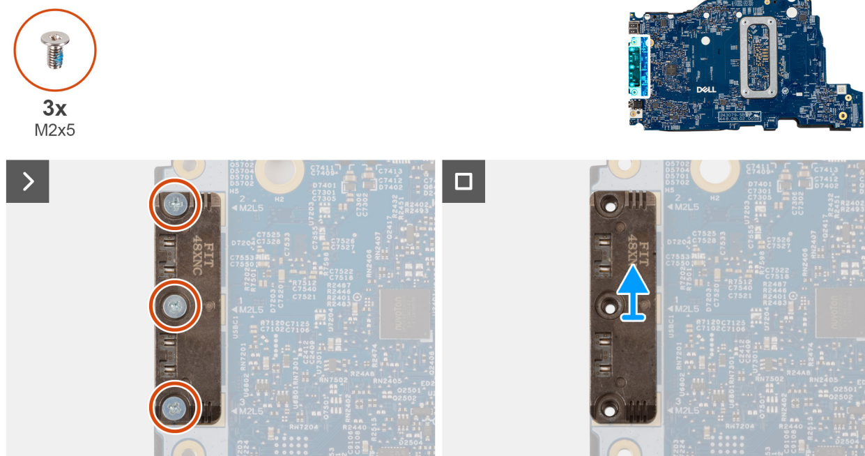
Obrázek 48. Demontáž modulu USB Type-C
