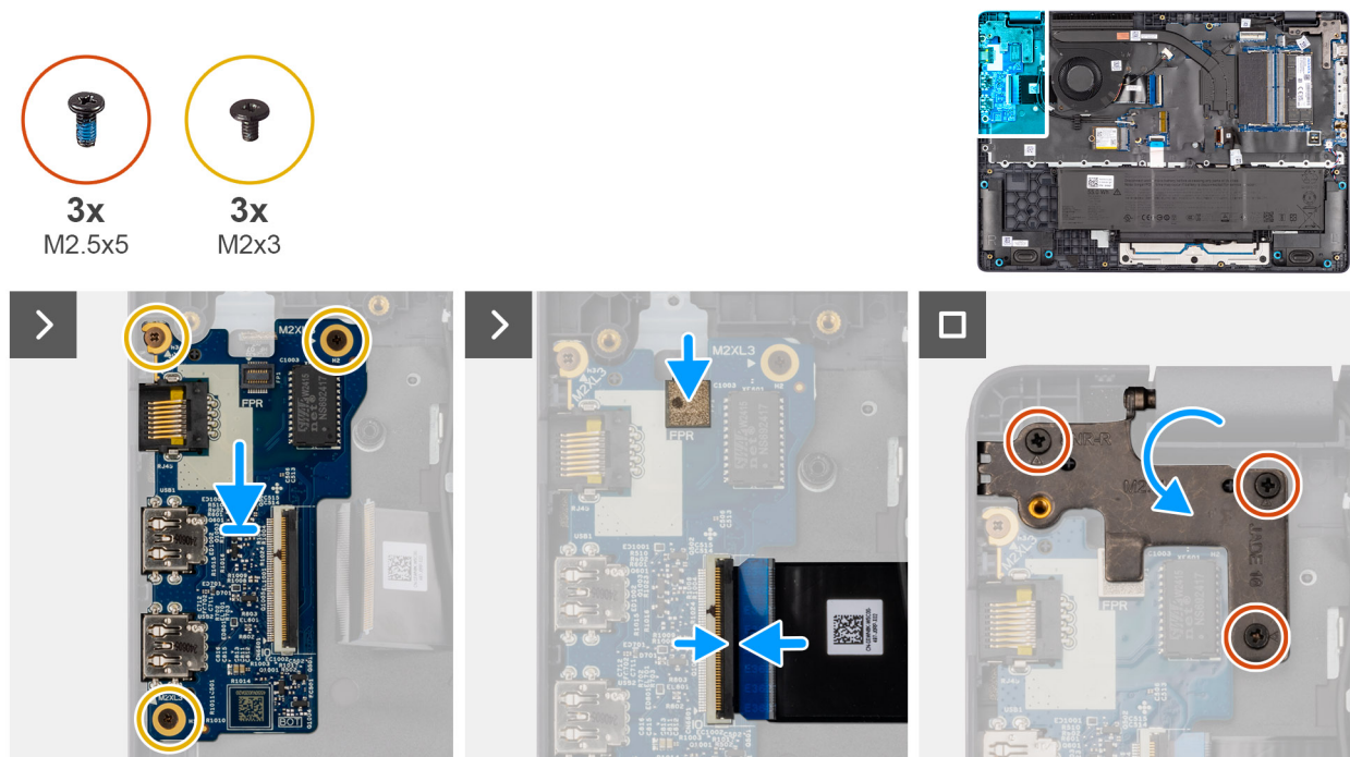
Obrázek 37. Vložení desky I/O
