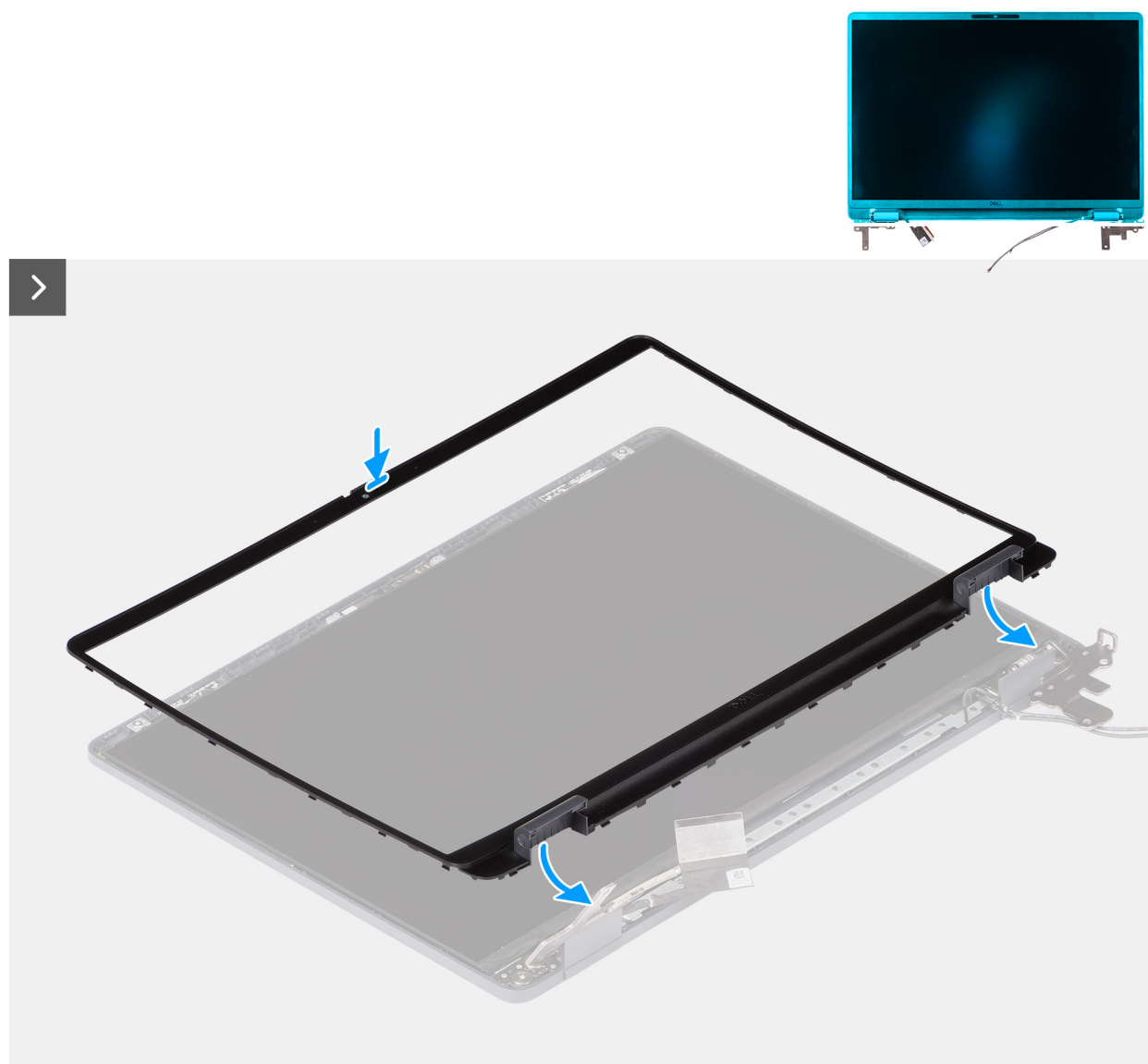
Obrázek 72. Montáž čelního krytu displeje
