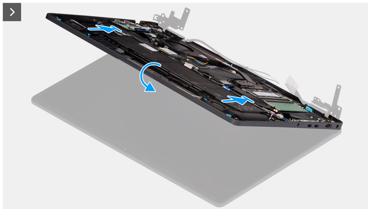
Obrázek 65. Montáž sestavy displeje
