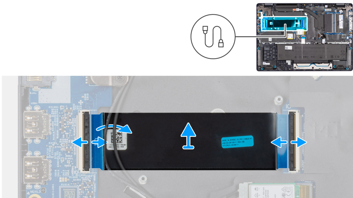
Obrázek 38. Demontáž kabelu FPC desky I/O
