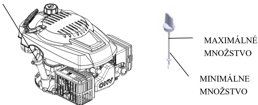
VIEČKO PLNIEHO OTVORU PRE OLEJ/OLEJOVÁ MIERKA
