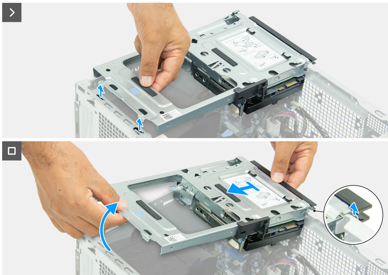
Obrázek 43. Demontáž diskové pozice
