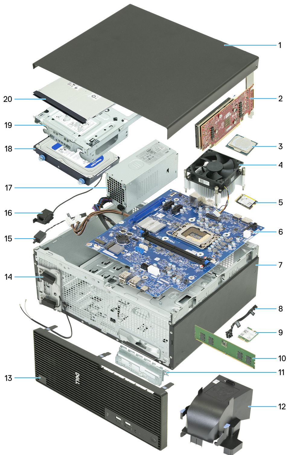
Obrázek 10. Hlavní komponenty počítače Dell Pro Tower QCT1250
