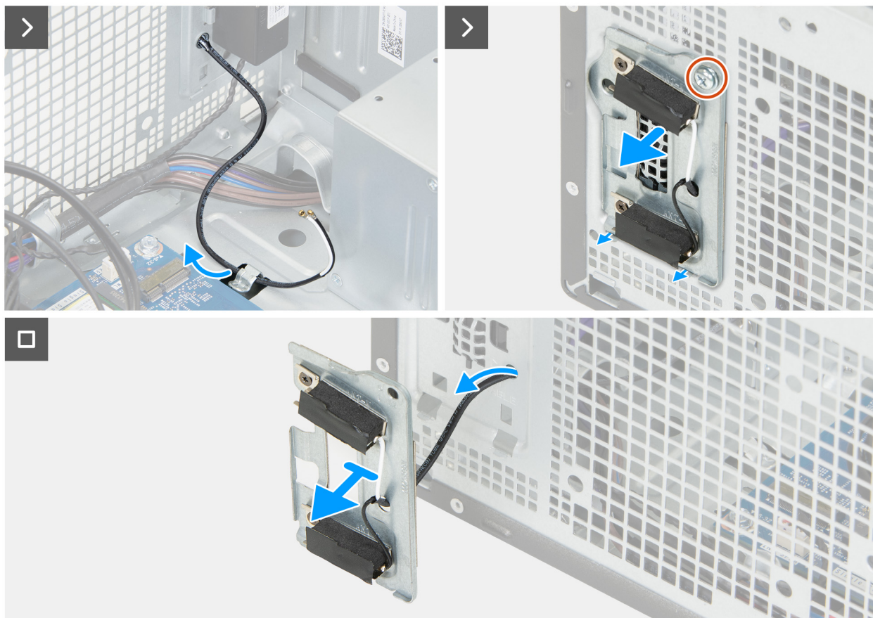
Obrázek 60. Demontáž anténních modulů
