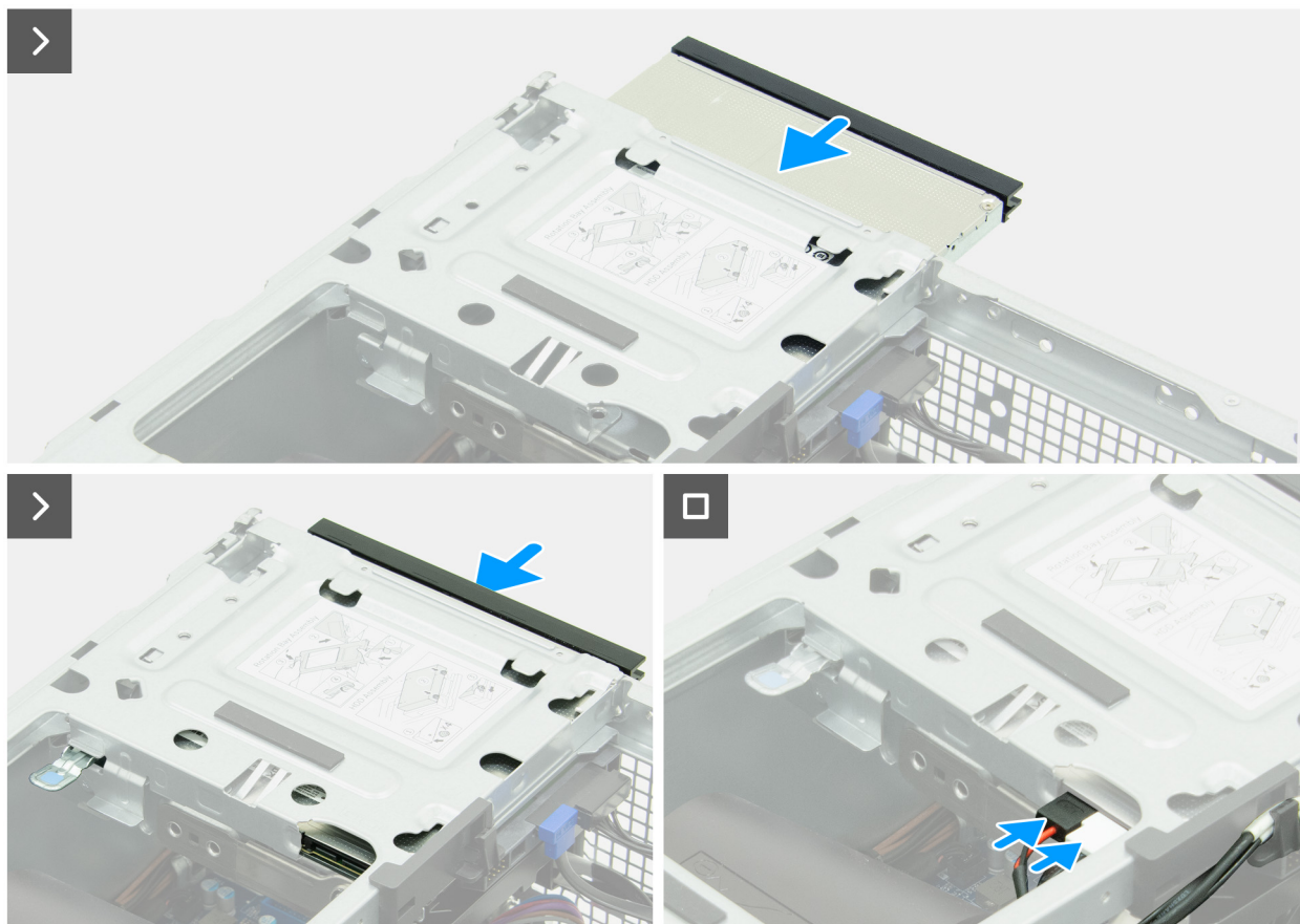
Obrázek 41. Montáž optické jednotky
