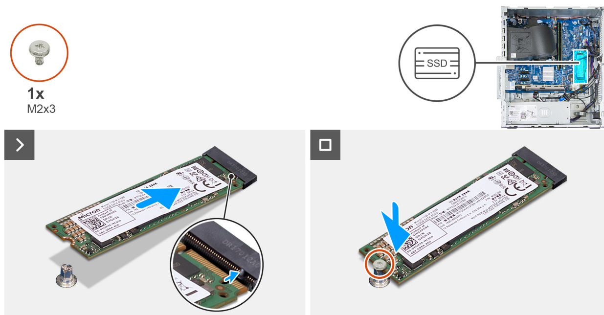
Obrázek 32. Montáž disku SSD M.2 2280
