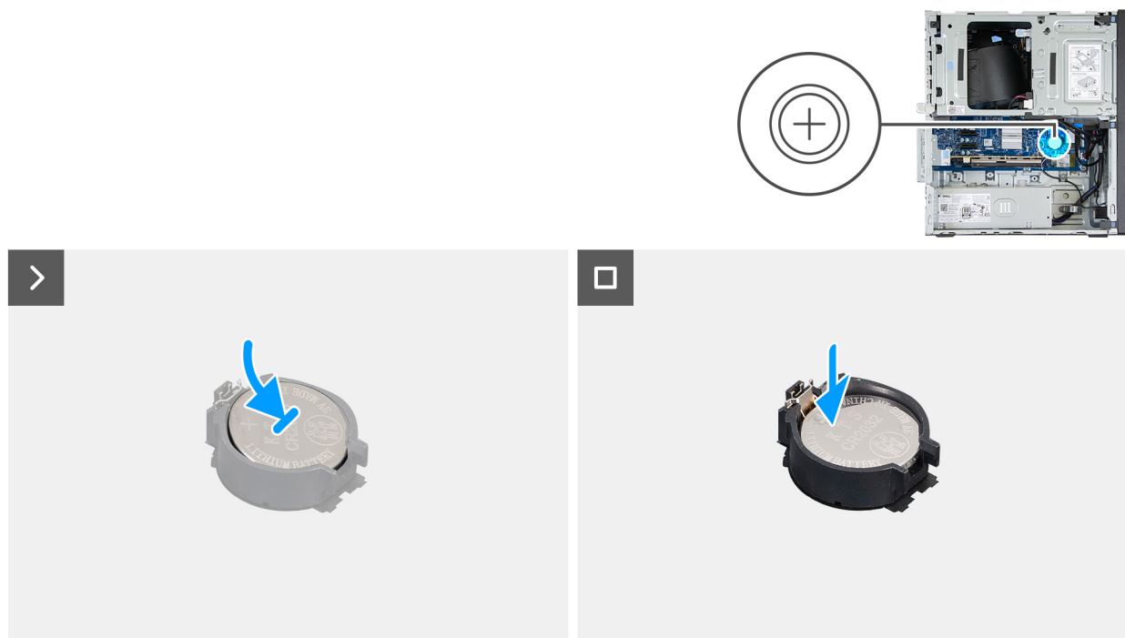
Obrázek 20. Montáž knoflíkové baterie
