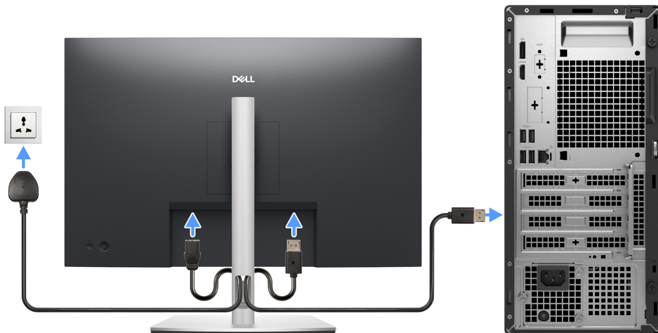
Obrázek 7. Připojení displeje
