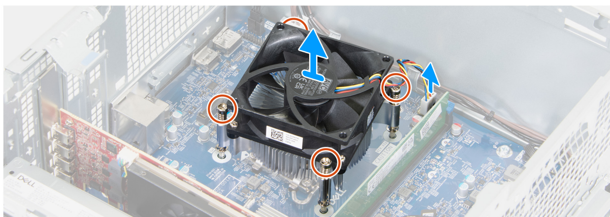
Obrázek 66. Demontáž sestavy ventilátoru a chladiče procesoru
