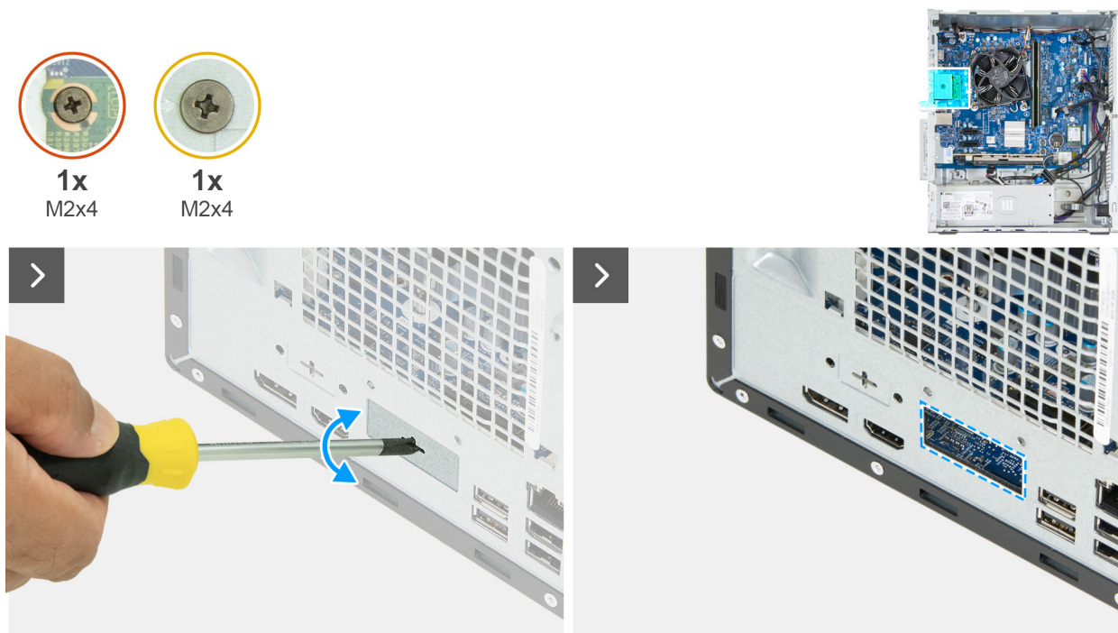
Obrázek 55. Montáž modulu volitelného portu
