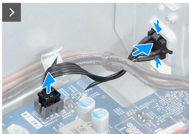
Obrázek 50. Demontáž vypínače
