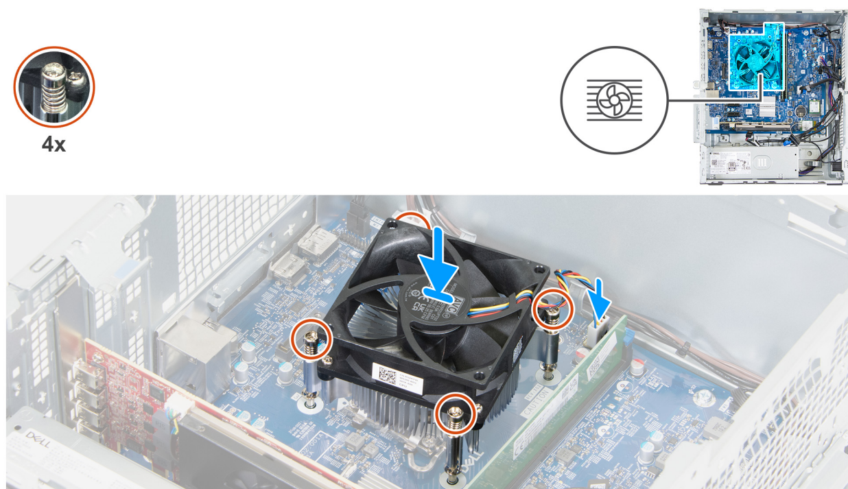
Obrázek 67. Montáž sestavy ventilátoru a chladiče procesoru
