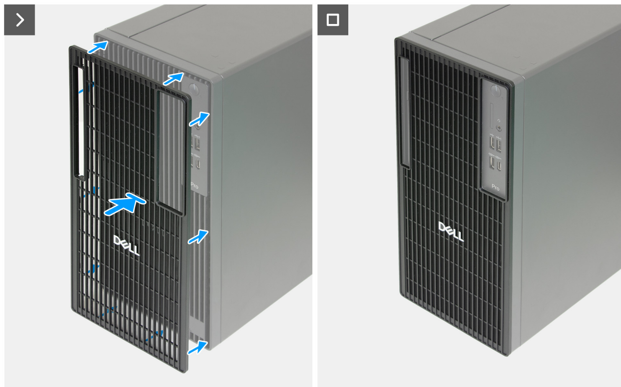
Obrázek 22. Montáž prachového filtru
