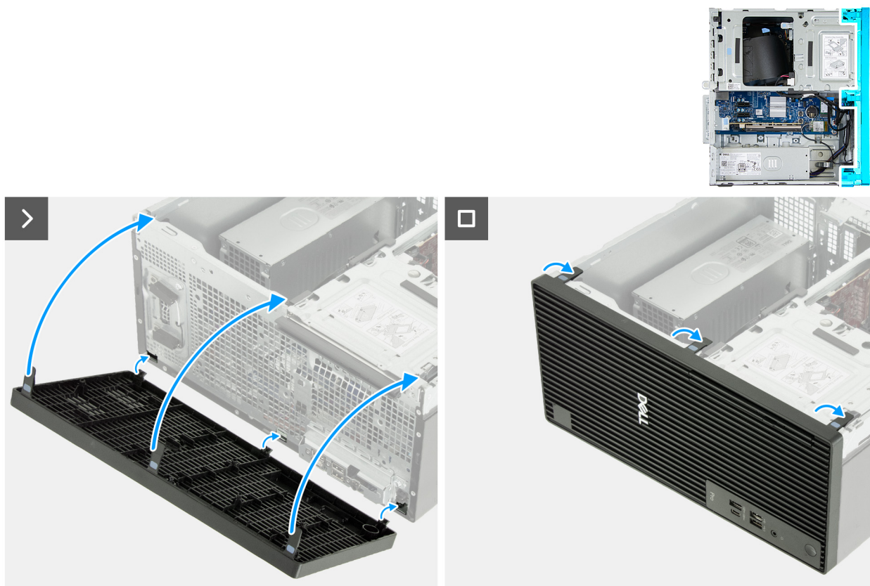
Obrázek 24. Montáž předního krytu
