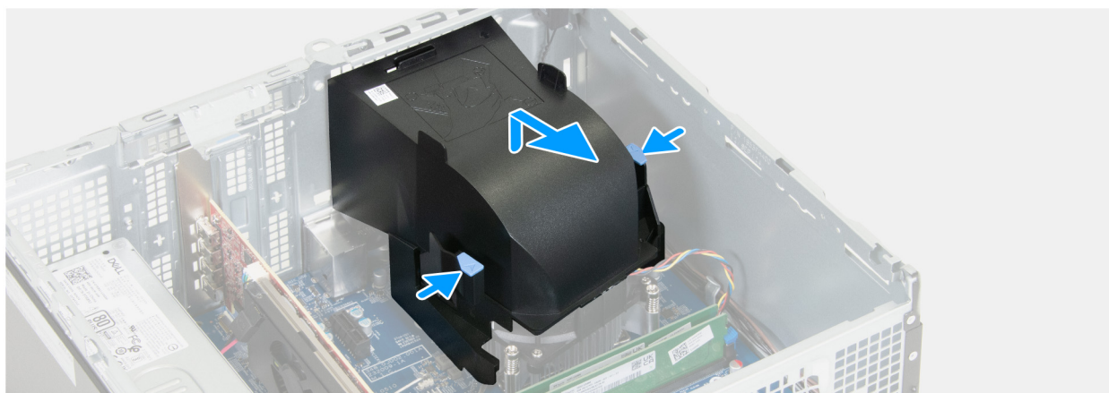
Obrázek 52. Obrázek: Demontáž krytu ventilátoru
