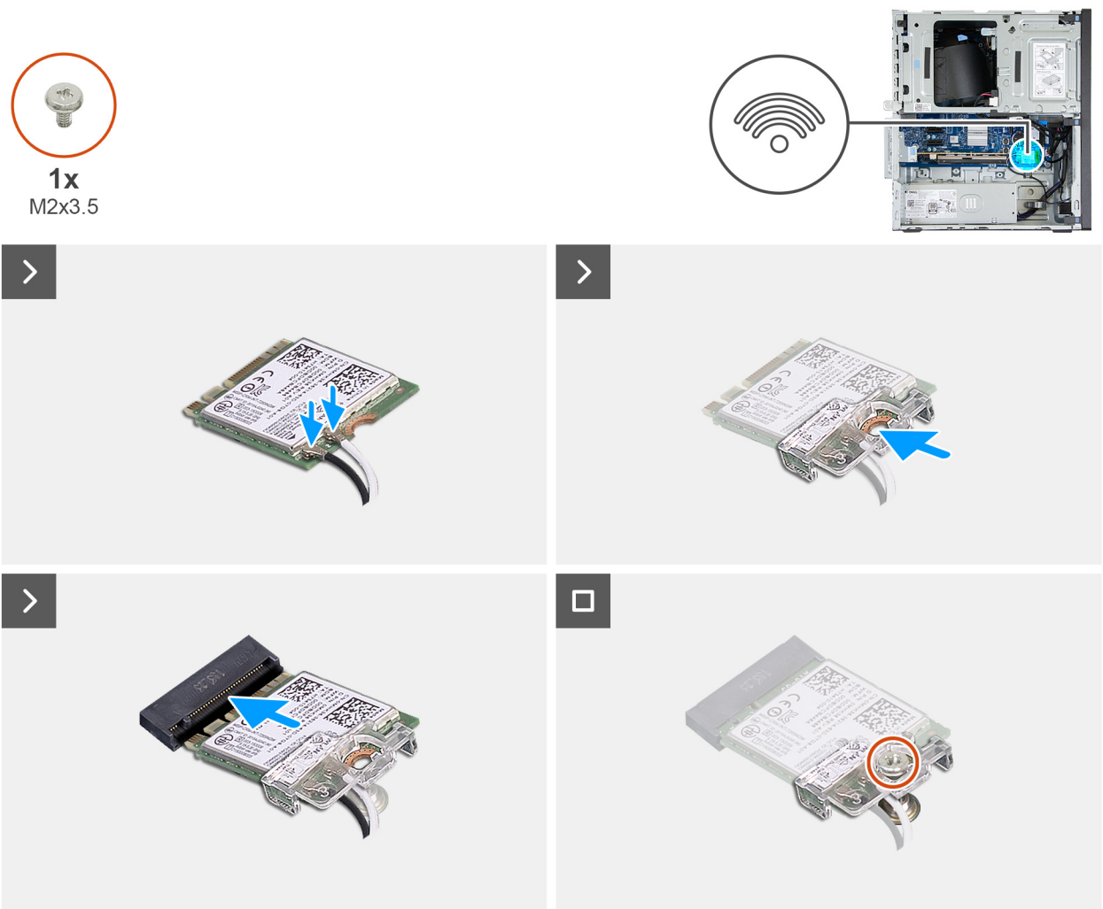
Obrázek 37. Montáž bezdrátové karty
