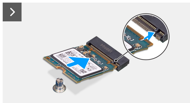
Obrázek 30. Montáž disku SSD M.2 2230
