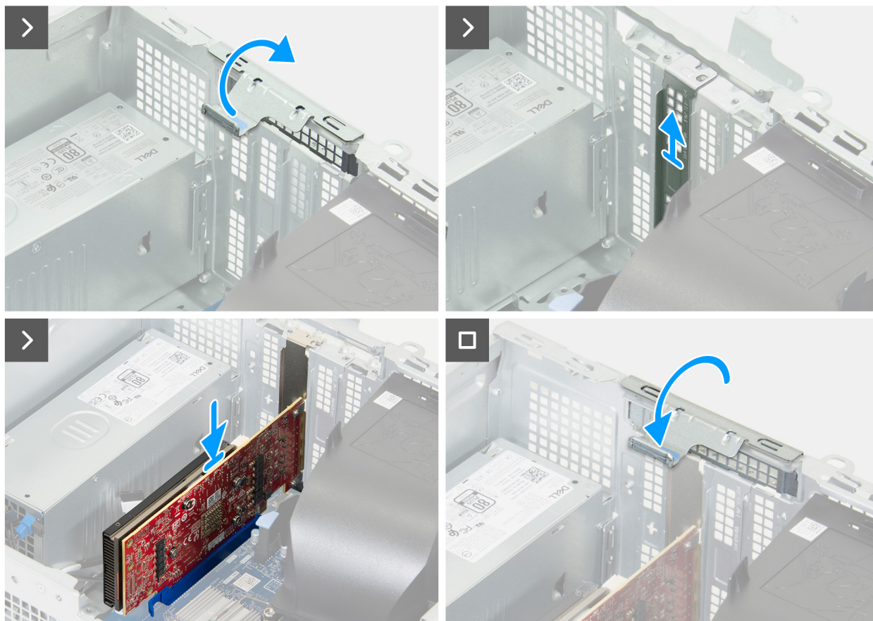
Obrázek 35. Montáž grafické karty
