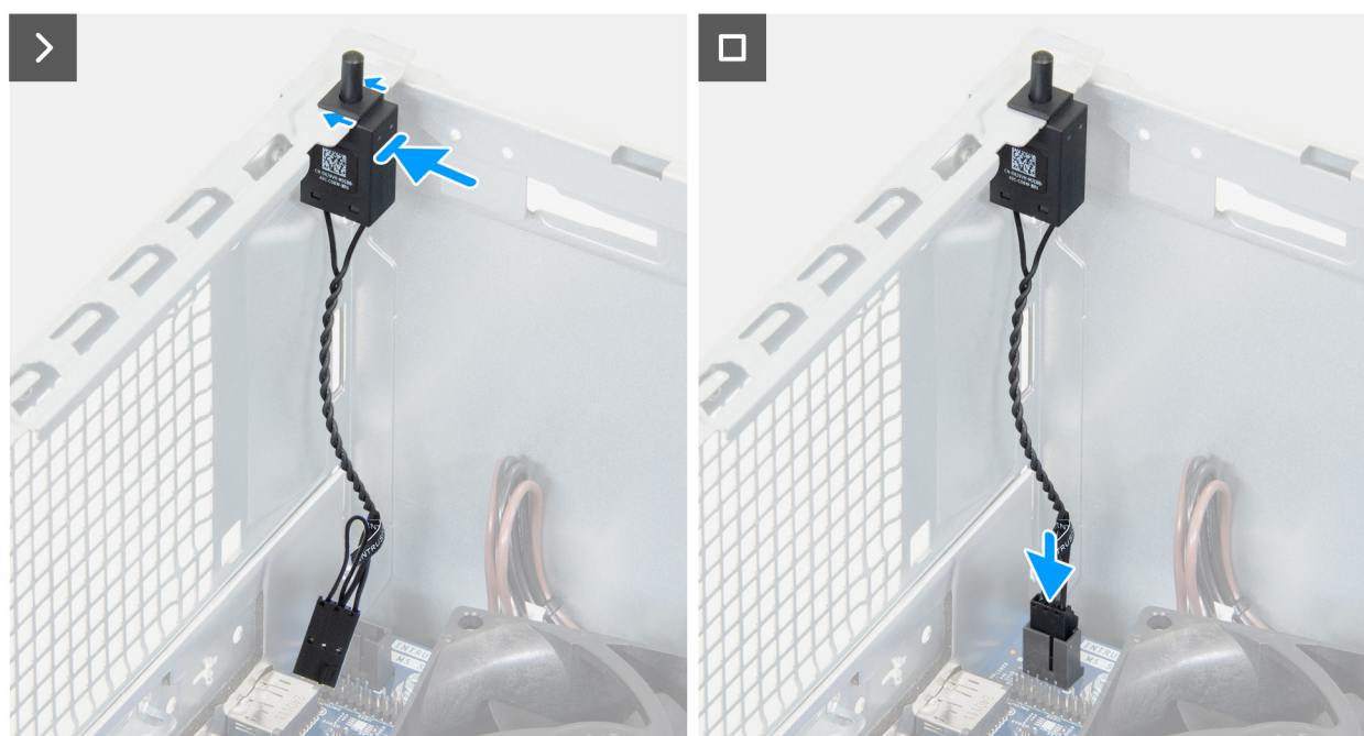
Obrázek 49. Montáž spínače detekce vniknutí do šasi
