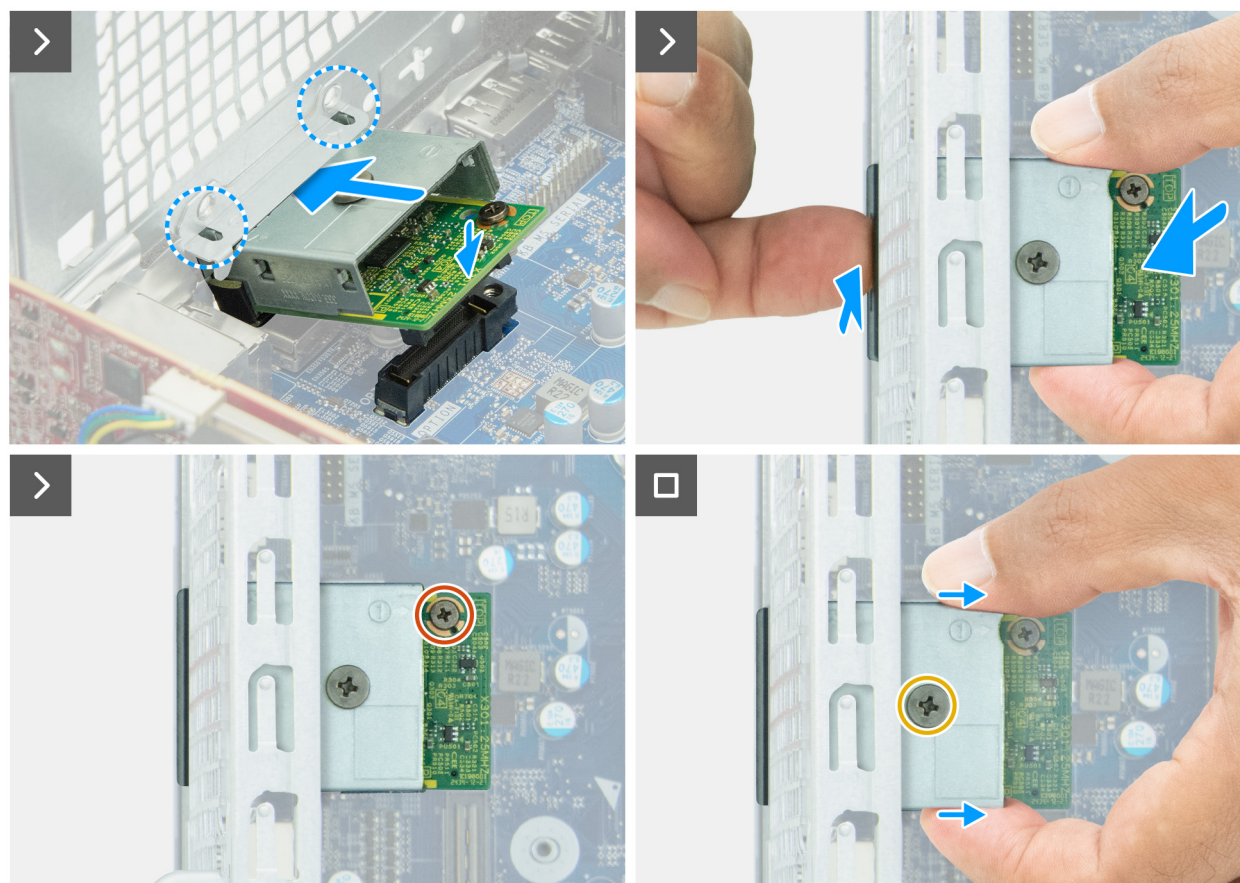
Obrázek 56. Montáž modulu volitelného portu
