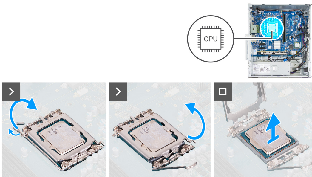
Obrázek 68. Demontáž procesoru
