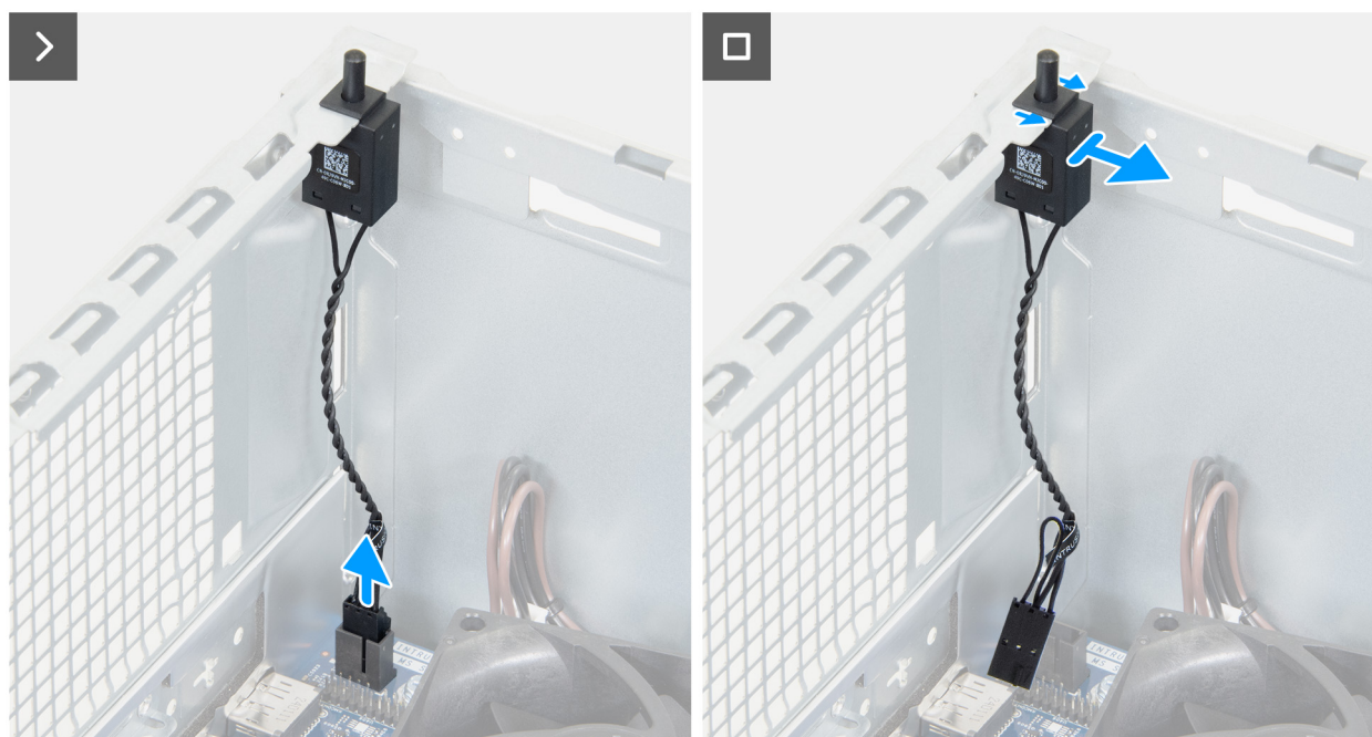
Obrázek 48. Demontáž spínače detekce vniknutí do šasi
