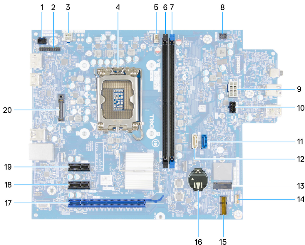
Obrázek 75. Popisky základní desky
