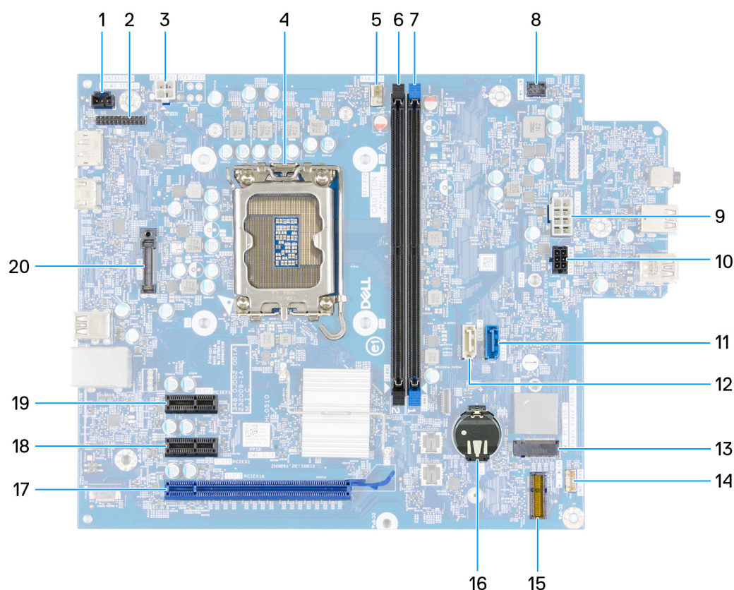
Obrázek 70. Popisky základní desky
