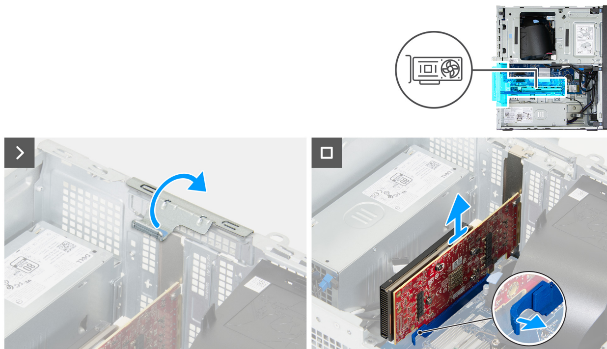
Obrázek 34. Demontáž grafické karty
