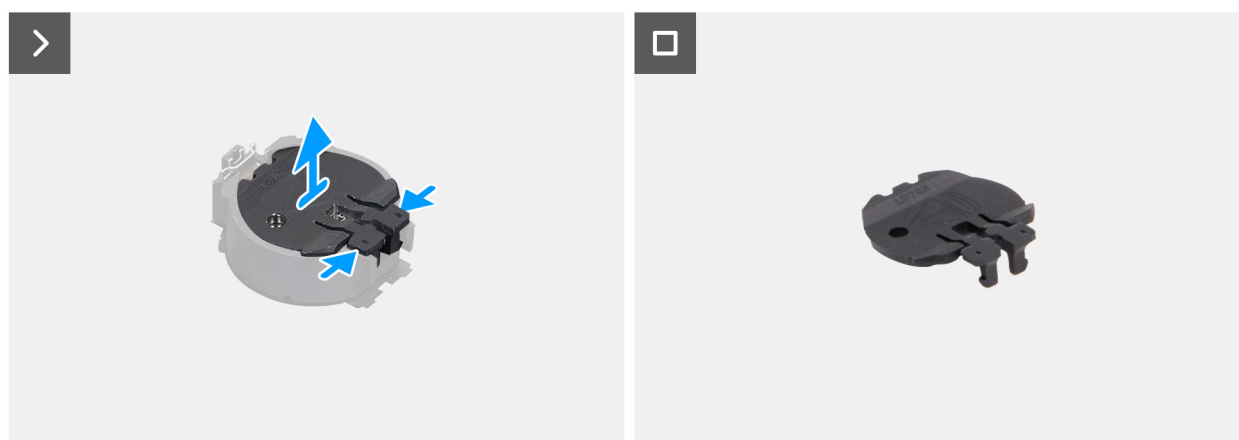
Obrázek 17. Demontáž krytu knoflíkové baterie
