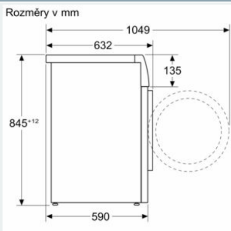
Rozměrové výkresy
